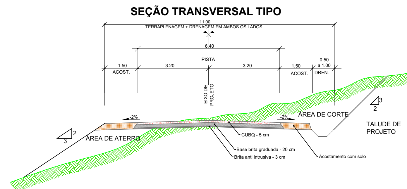
04 Seção Transversal Tipo Escala: 1/100
