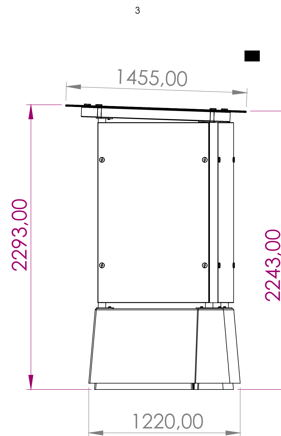
VISTA LATERAL
