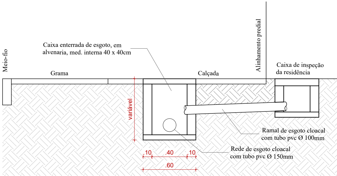
Detalhe 2 - Caixa e Ramal de Esgoto Cloacal Escala 1/25
