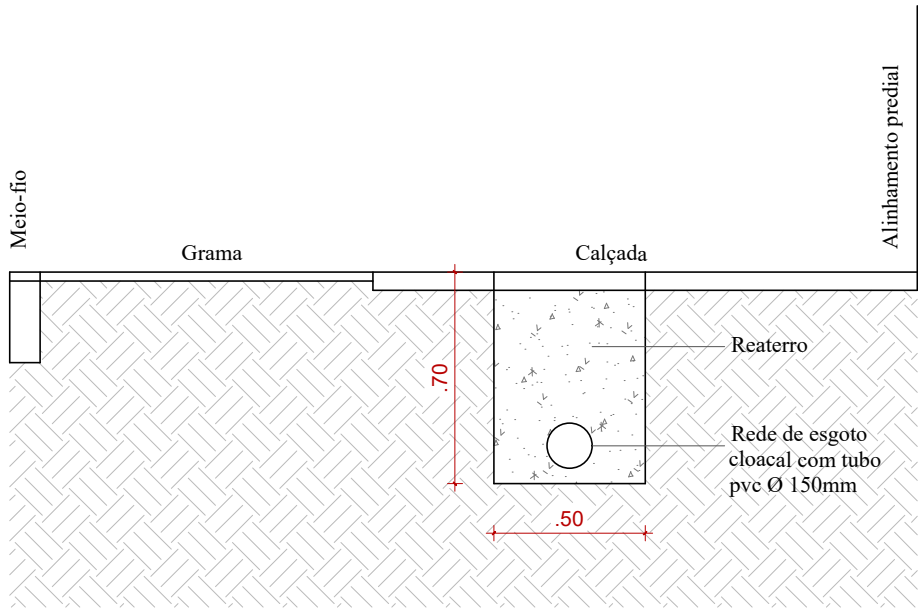
Detalhe 1 - Rede de Esgoto Cloacal Escala 1/25
