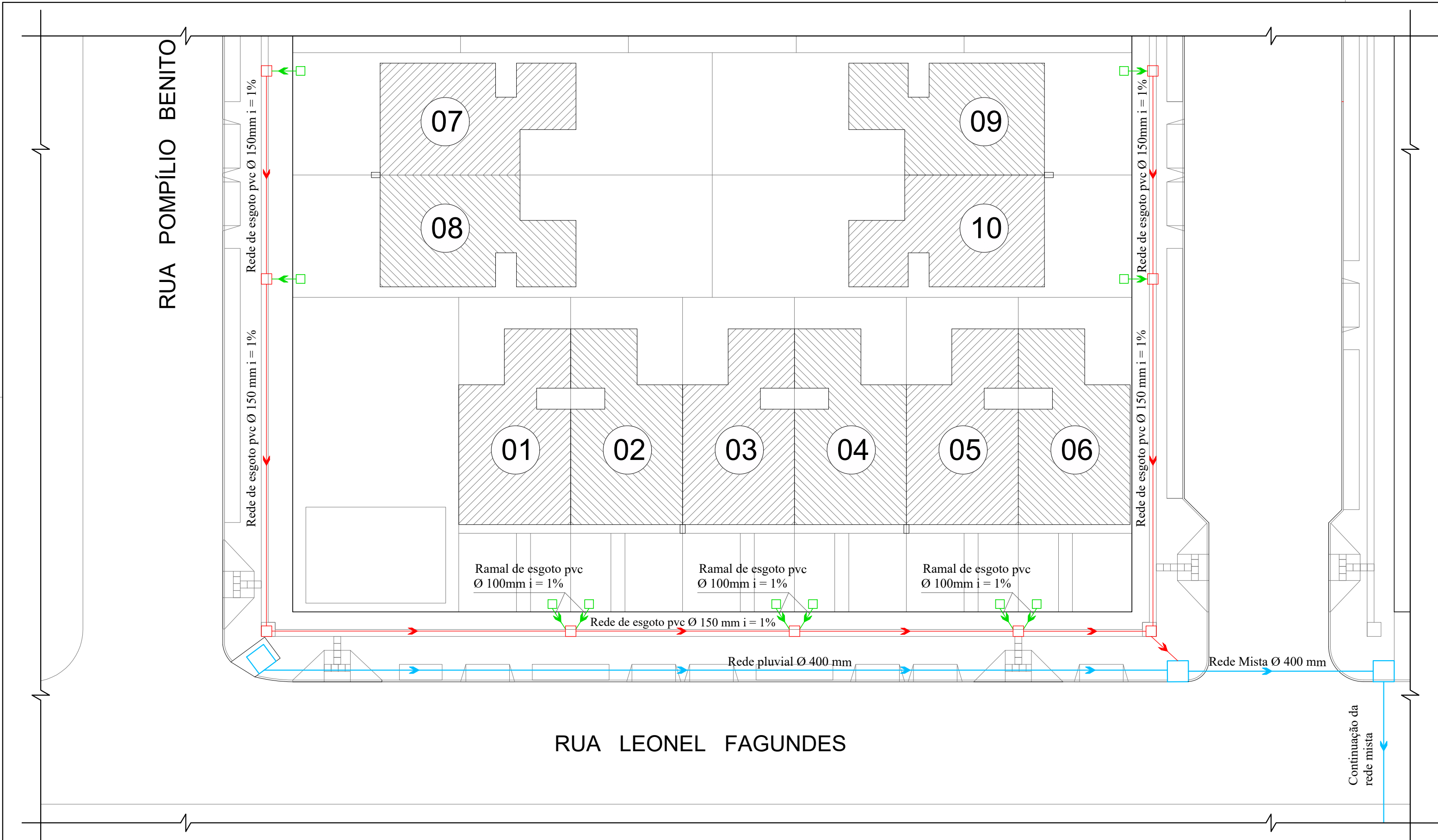
Planta de Drenagem Cloacal e Pluvial (Rede Mista) Escala 1/200
