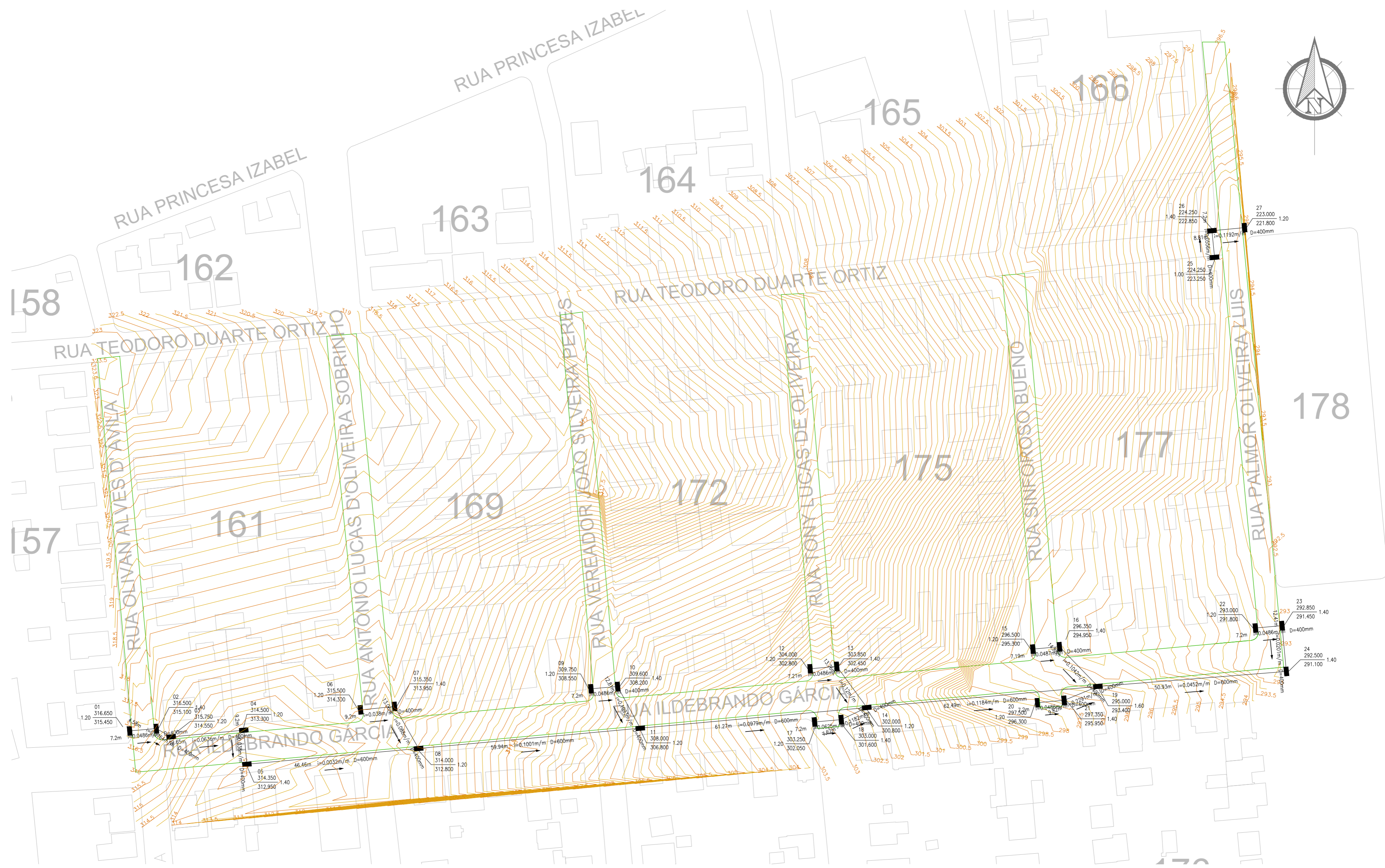
PLANTA PROJETO DE DRENAGEM Esc.: 1/750
