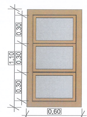
Detalhe janela
