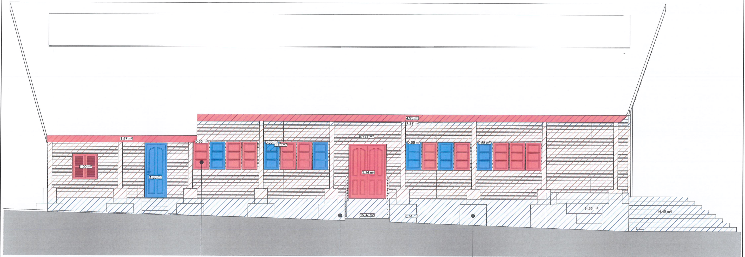
Fachada de Intervenção Esc. 1:75
