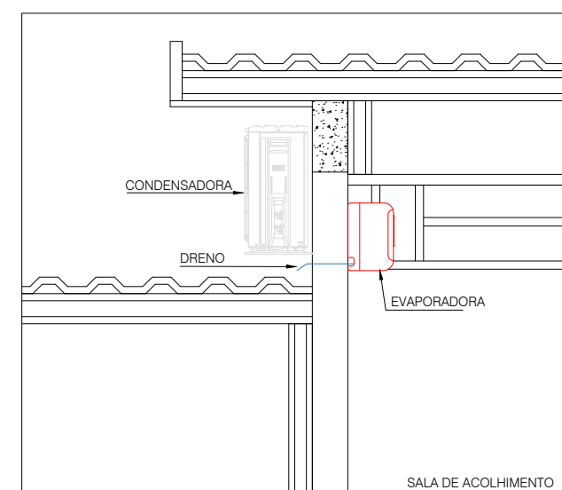
3 DETALHE 8 - INSTALAÇÃO AR CONDICIONADO SALA DE ACOLHIMENTO Esc.: 1/20
