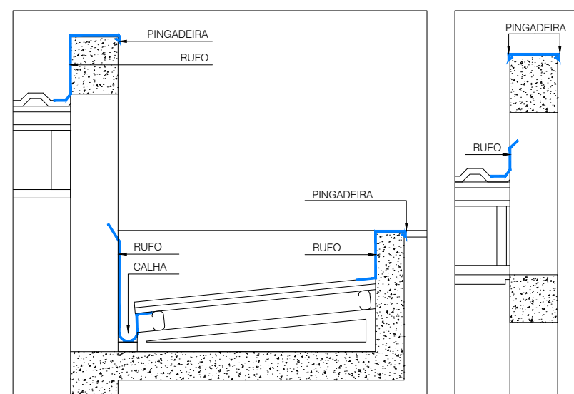
2 DETALHE 3 - RUFOS COBERTURA Esc.: 1/20
