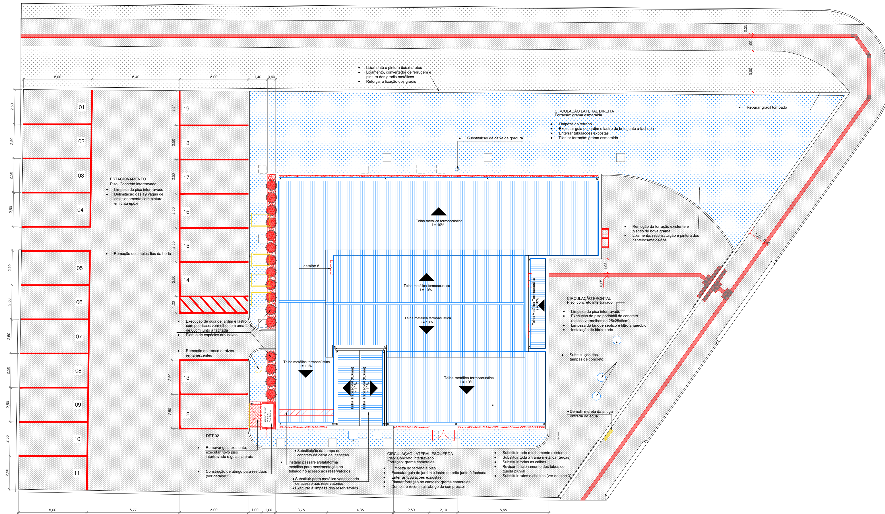
1 PLANTA DE IMPLANTAÇÃO E COBERTURA - INTERVENÇÕES Esc.: 1/100
