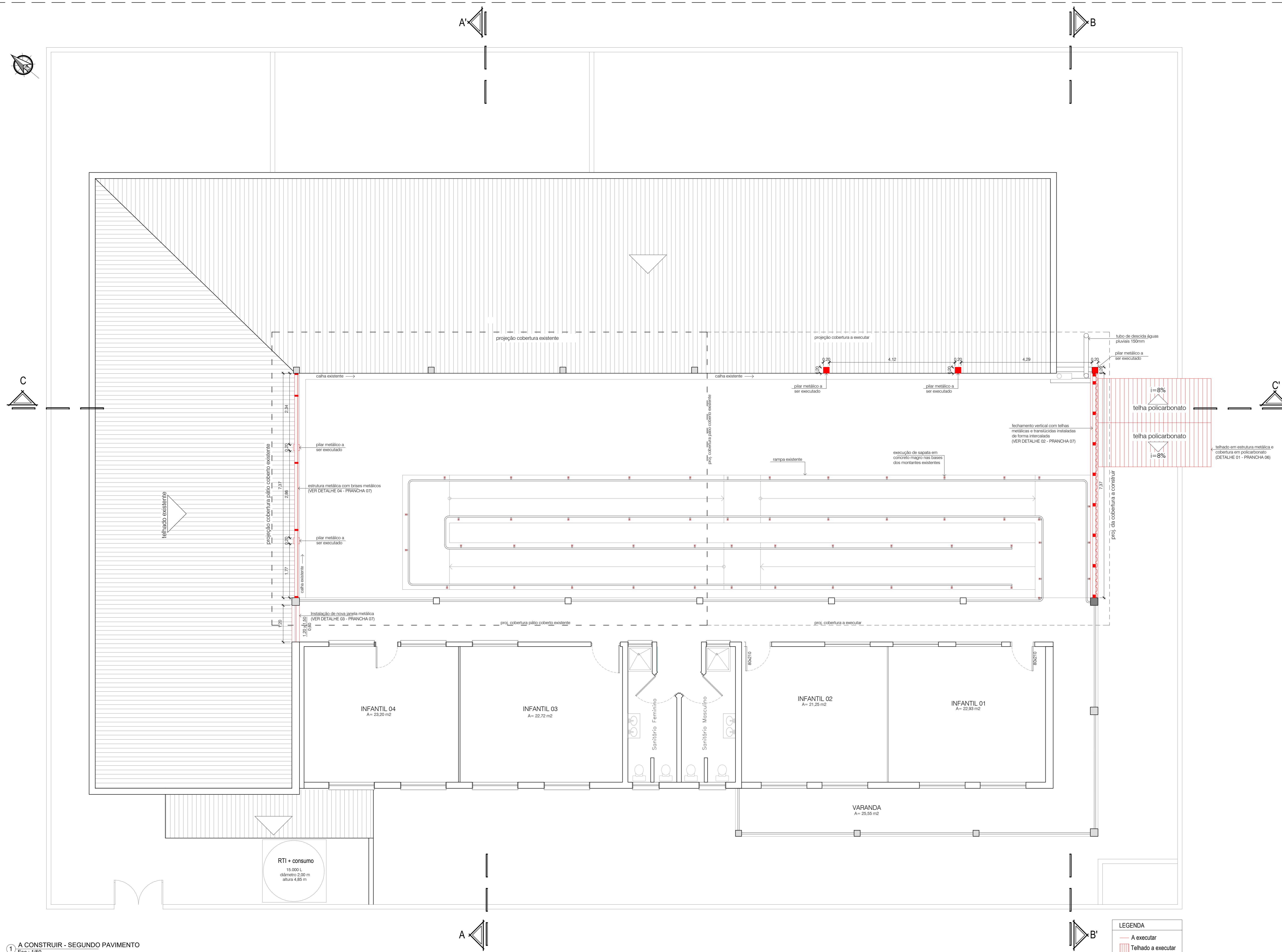
1 A CONSTRUIR - SEGUNDO PAVIMENTO Esc.: 1/50
