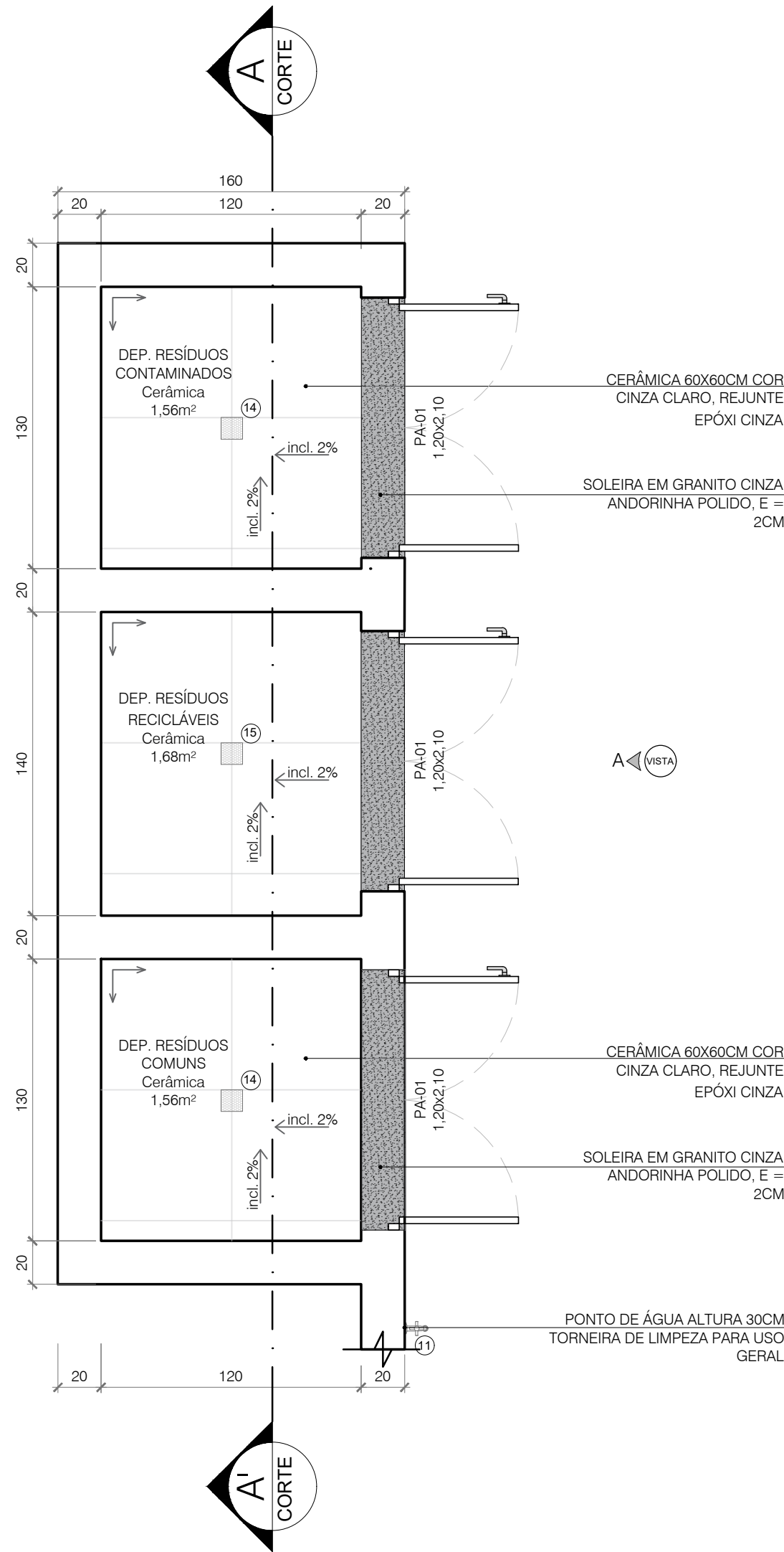
1 PLANTA BAIXA RESÍDUOS Esc.: 1/25
