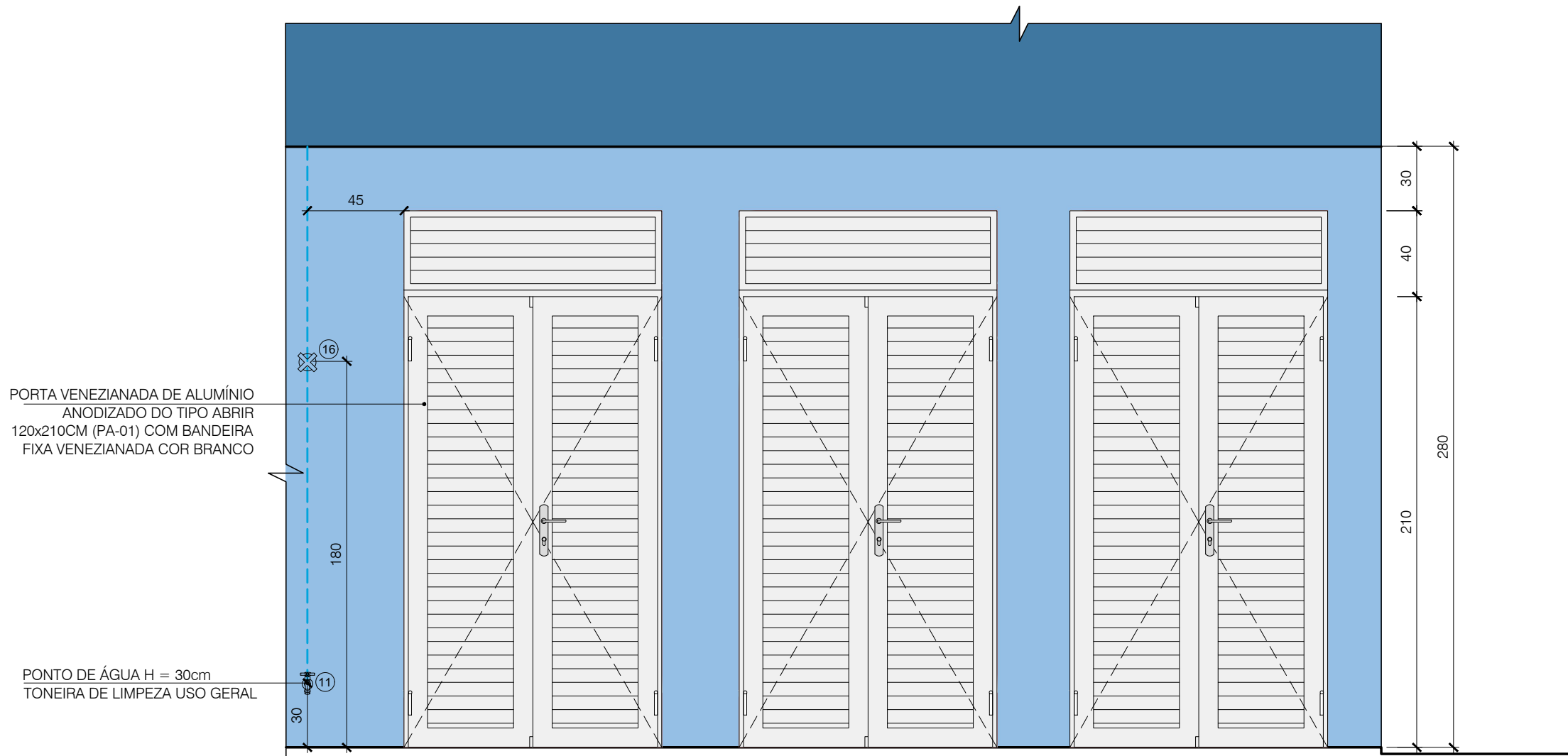
3 VISTA A - RESÍDUOS Esc.: 1/25
