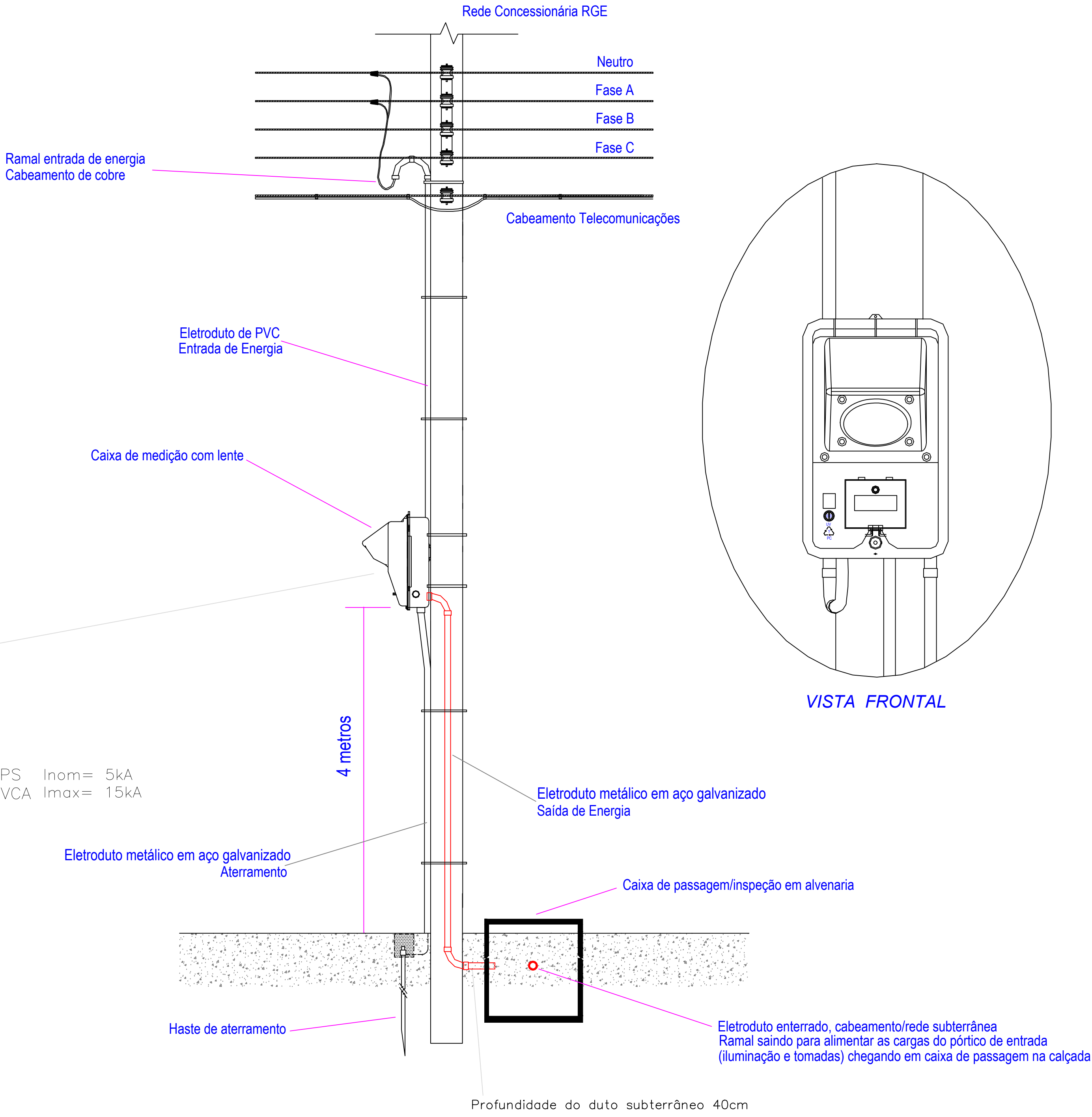
DETALHE PROTEÇÕES CAIXA MEDIÇÃO:
