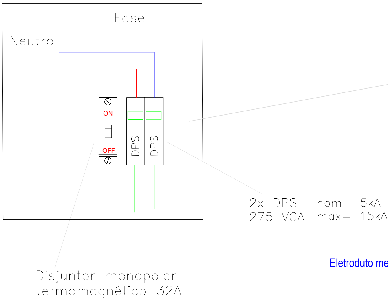
DETALHE PROTEÇÕES CAIXA MEDIÇÃO:
