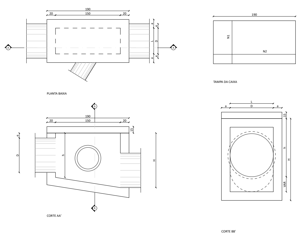
CAIXA DE LIGAÇÃO E PASSAGEM - CLP ESCALA 1:50
