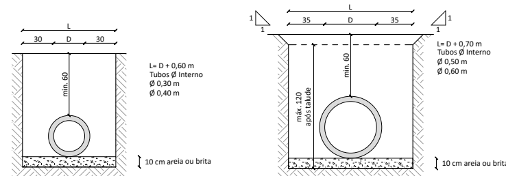
GABARITOS DE ESCAVAÇÃO ESCALA 1:50
