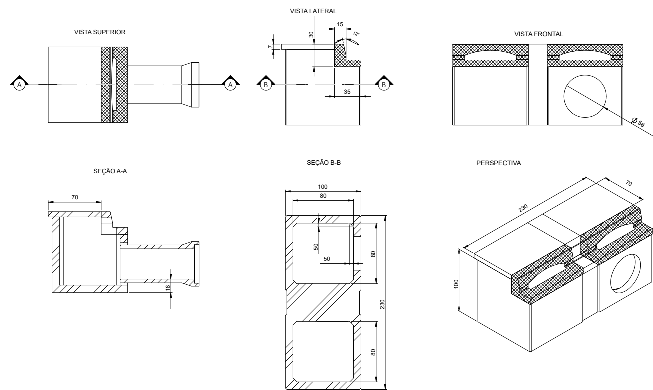
BOCA DE LOBO DUPLA - BLD ESCALA 1:50
