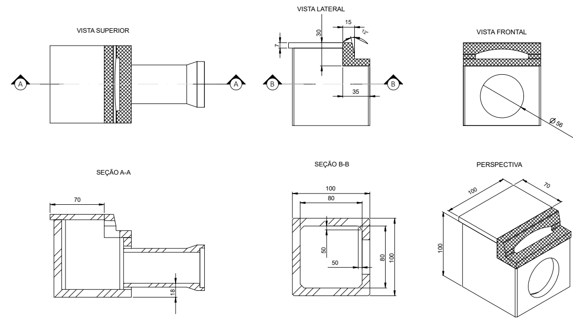
BOCA DE LOBO SIMPLES - BLS ESCALA 1:50
