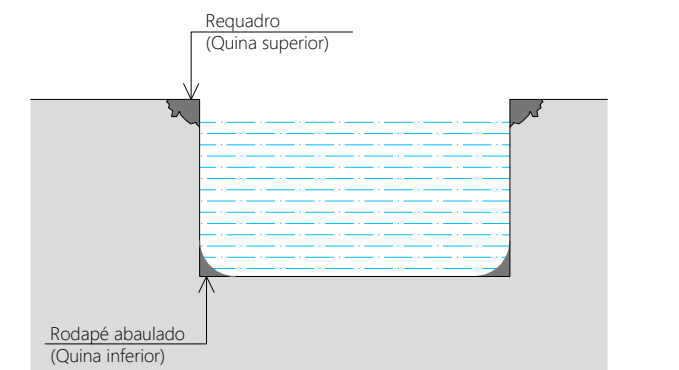
DETALHE TÍPICO ENCHIMENTOS SEM ESCALA
