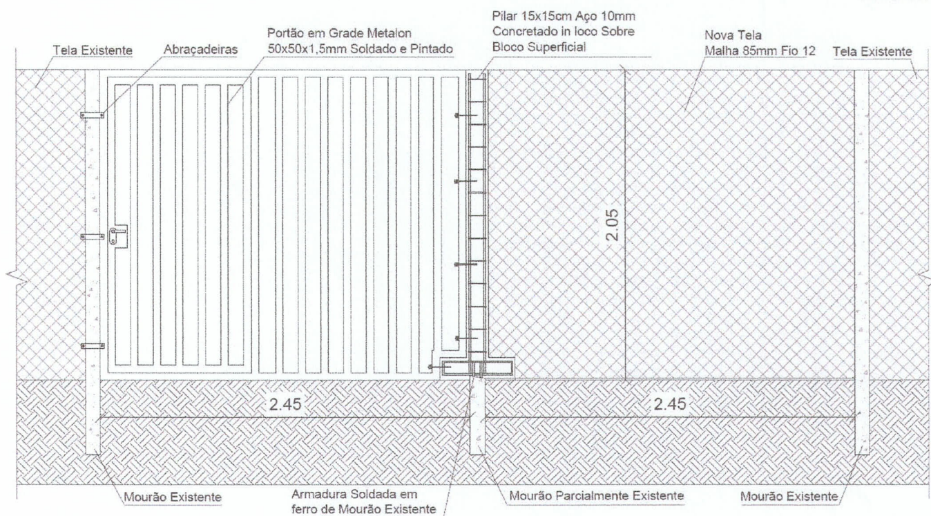
Figura 3 – Diagrama e especificações de montagem da estrutura
