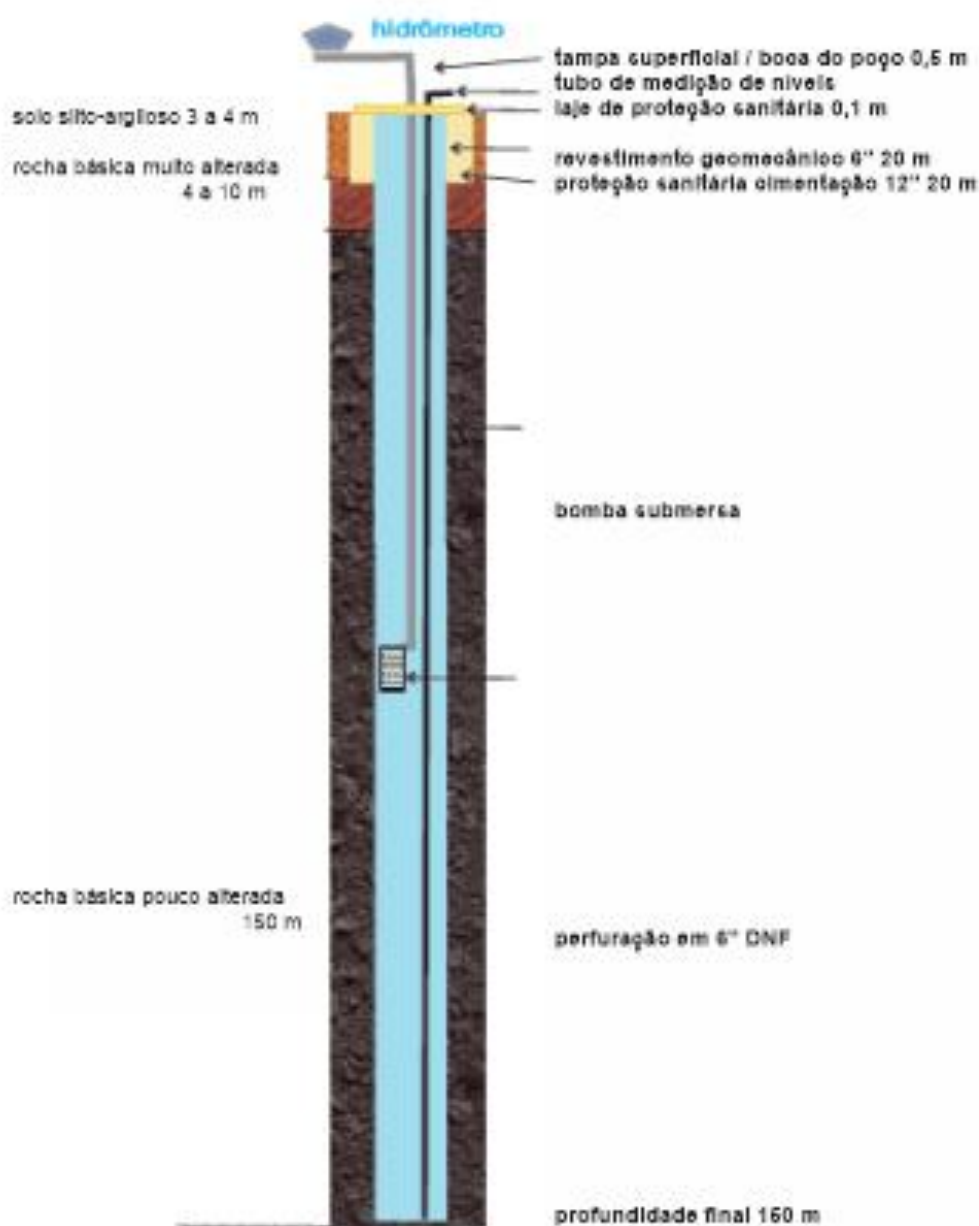
Figura 7 - Perfil esquemático previsto
