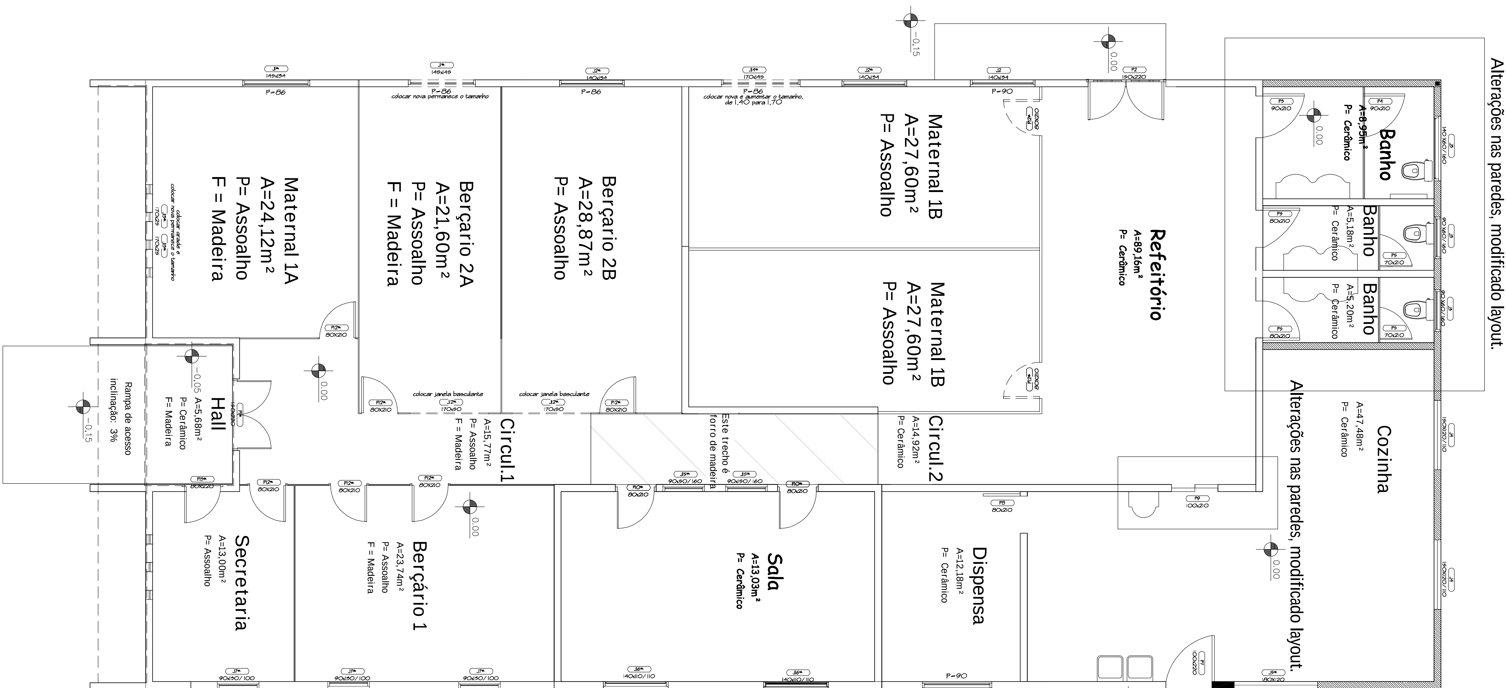
PLANTA BAIXA LAYOUT ATUAL ESC: 1/50
