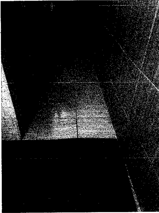
FOTO 01 – Piso estufado devido a dilatação e umidade.
