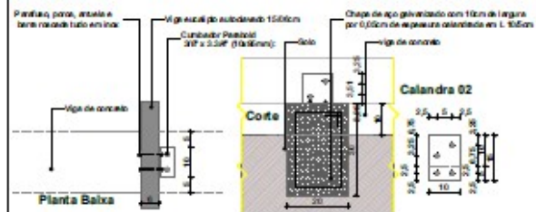
DET-FIXAÇÃO 1:10
