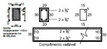
DET-VIGA 1:20
