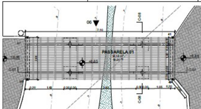
PASSARELA 01 1:50
