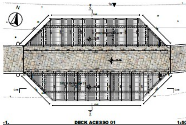
DECK ACESSO 01 1:50
