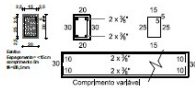
DET-VIGA 1:20
