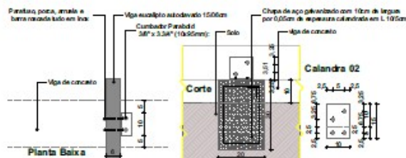
DET-FIXAÇÃO 1:10
