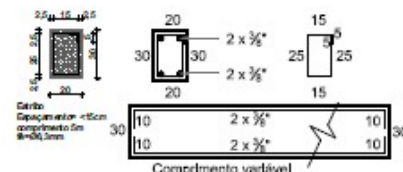
DET-VIGA 1:20
