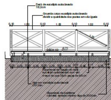
CORTE 17 1:50
