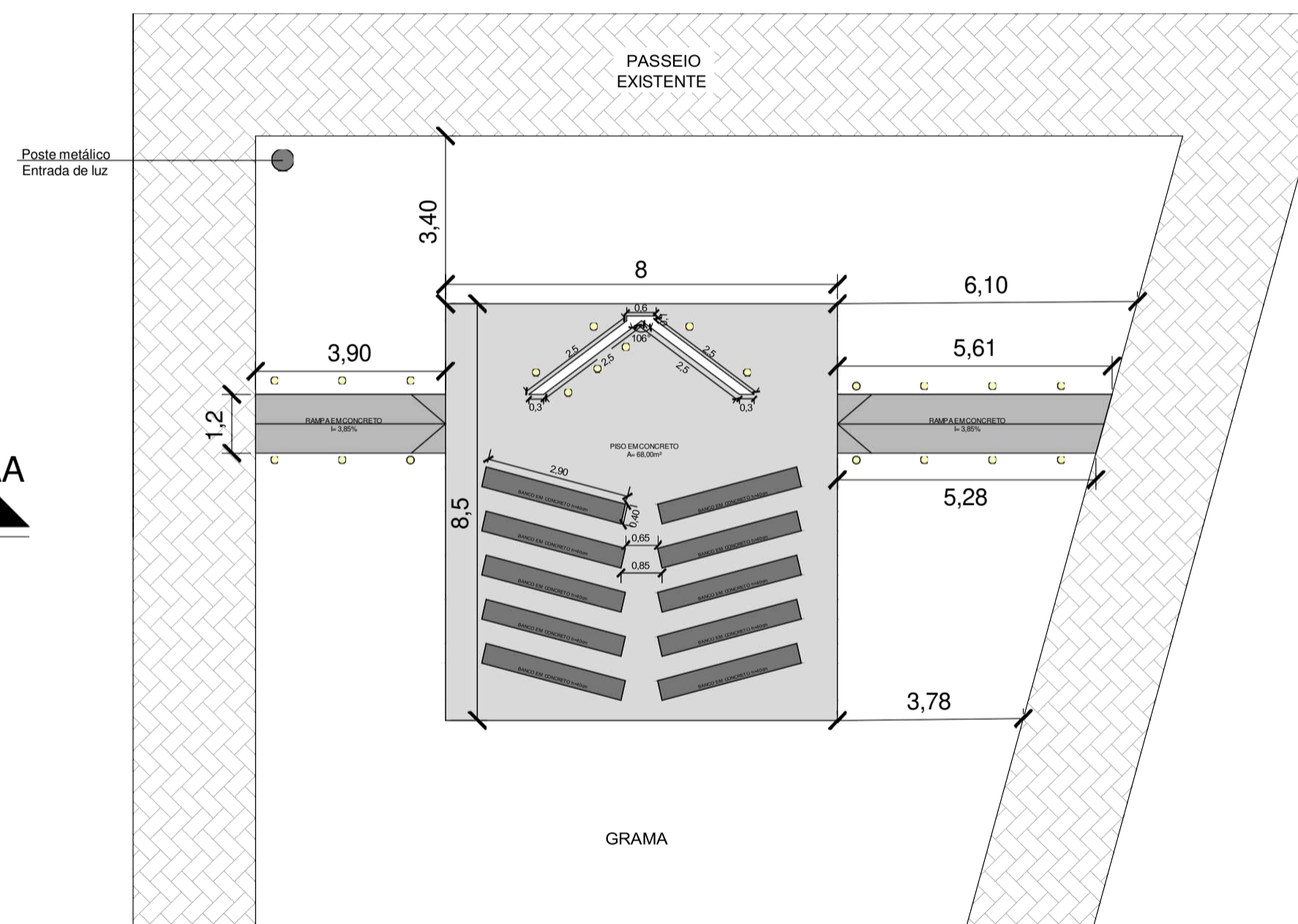
PLANTA BAIXA ESC: 1/75
