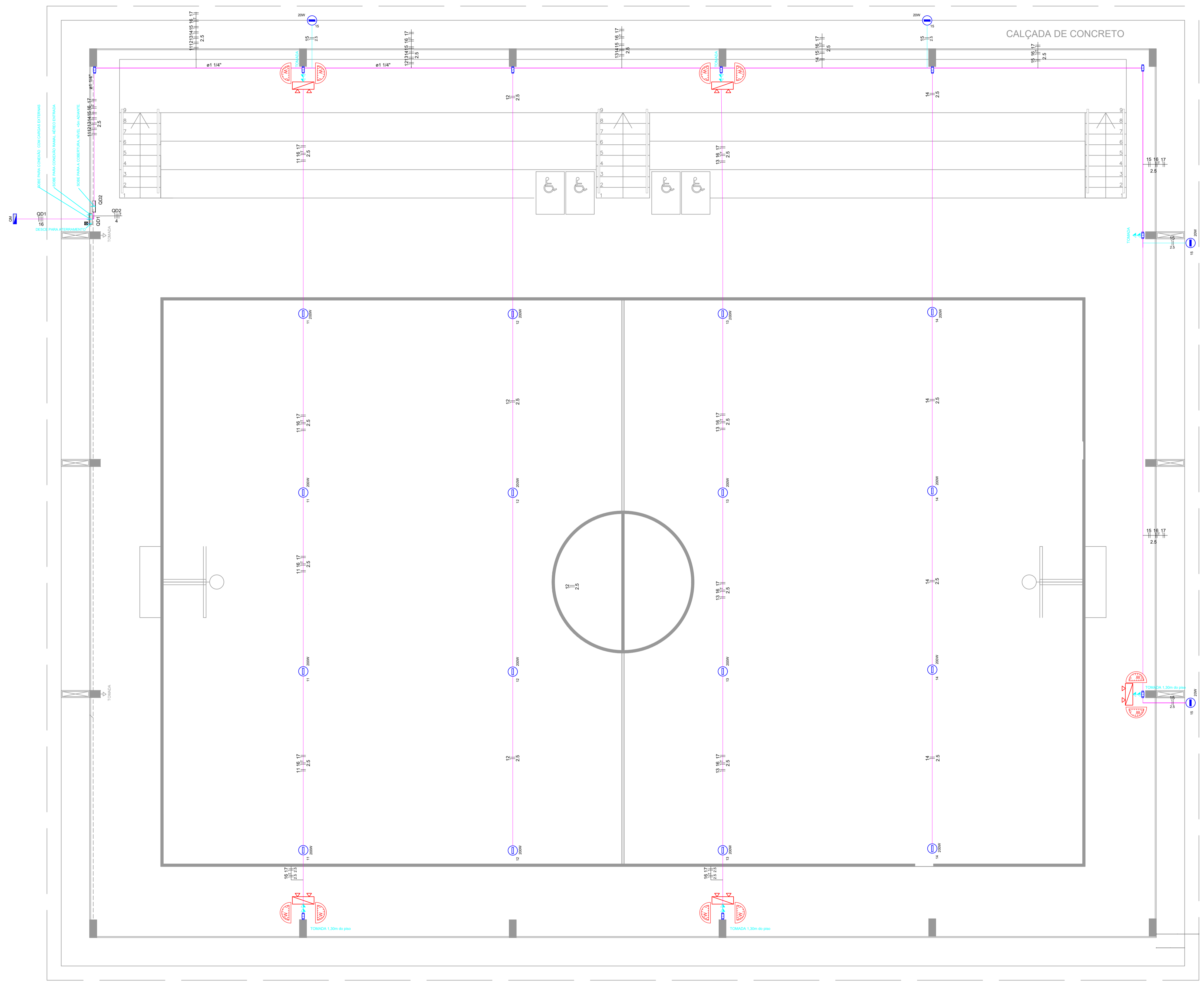
PROJEÇÃO DA COBERTURA 1 PROJETO ELÉTRICO ILUMINAÇÃO QUADRA ESCALA 1/50
