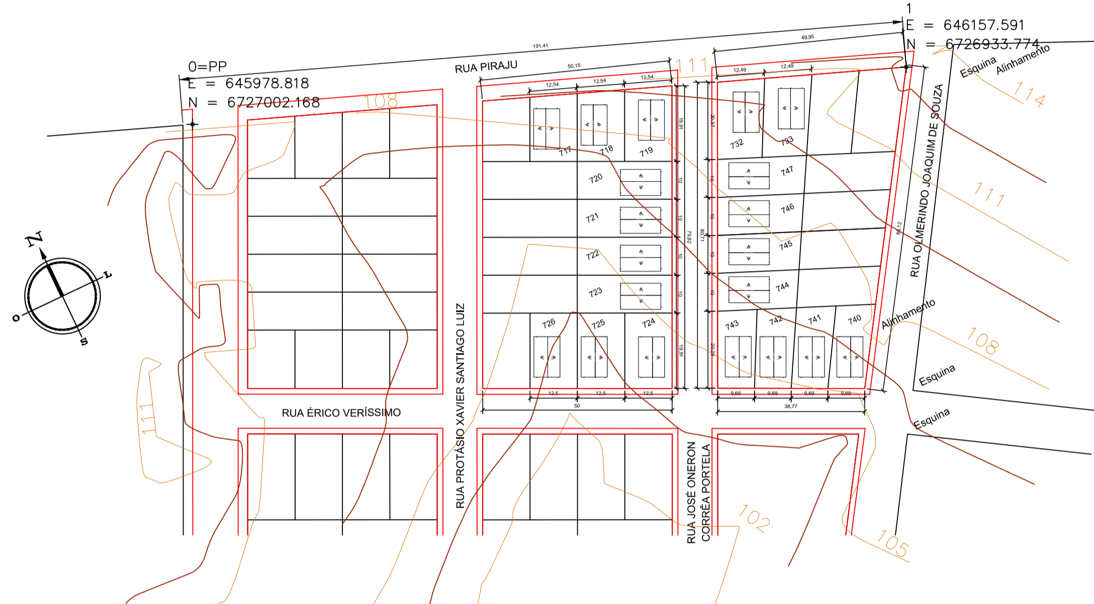
PLANTA DE SITUAÇÃO Esc.:1:1000
