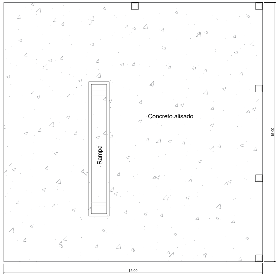
Planta de contraventamento da cobertura e locação dos pilares
