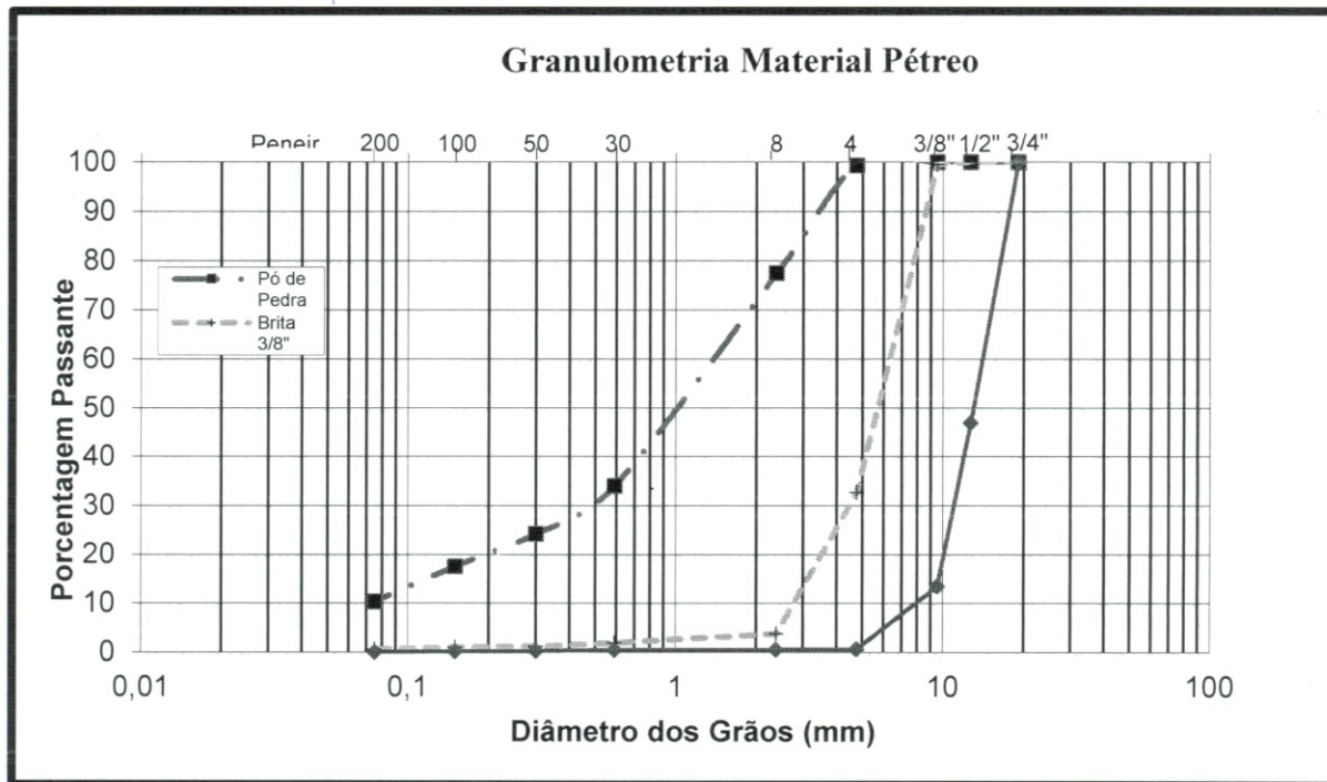
Curva Granulométrica dos materiais
