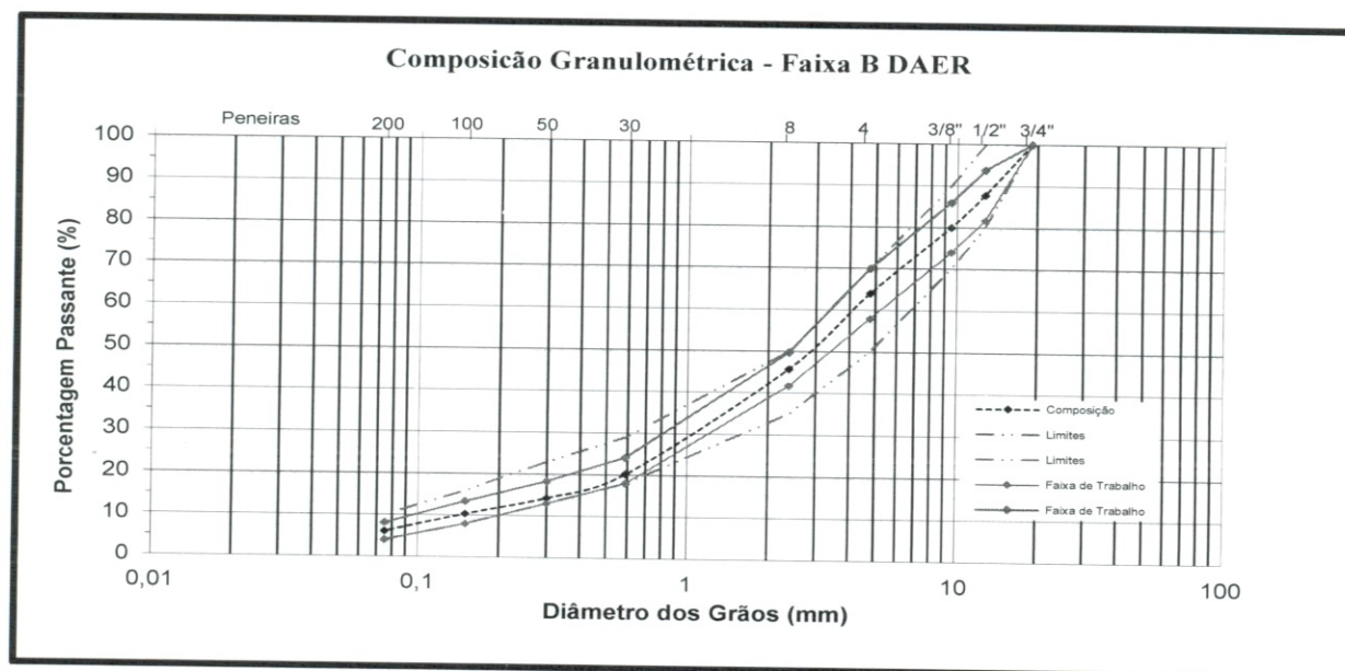
Curva granulométrica da mistura
