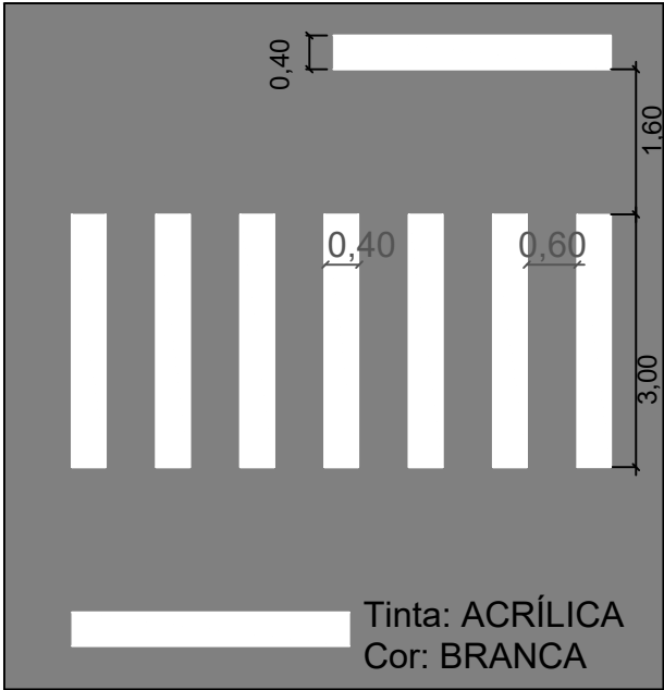
DETALHE: FAIXA DE SEGURANÇA
