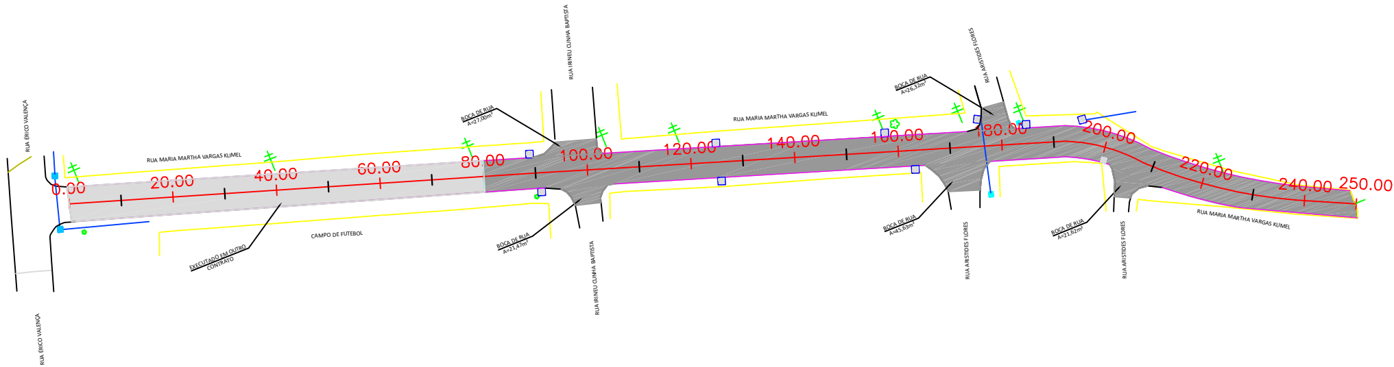
PLANTA BAIXA - PAVIMENTAÇÃO ESCALA: 1/1000
