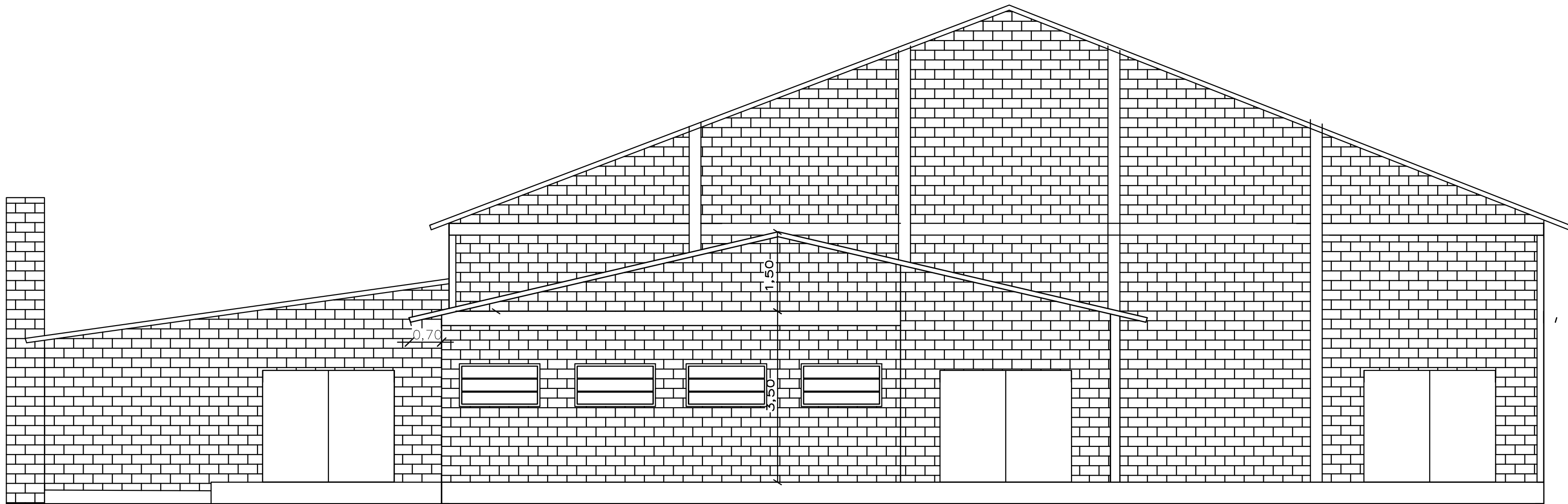
FACHADA FRONTAL
