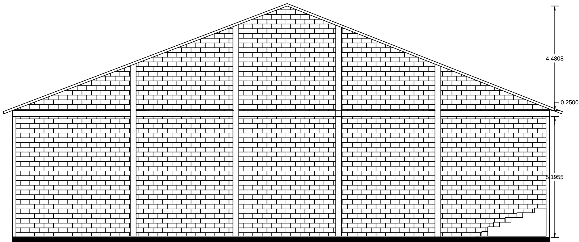
CORTE B-B
