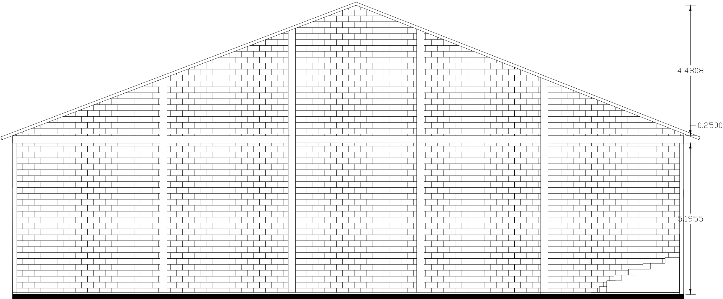
CORTE C-C
