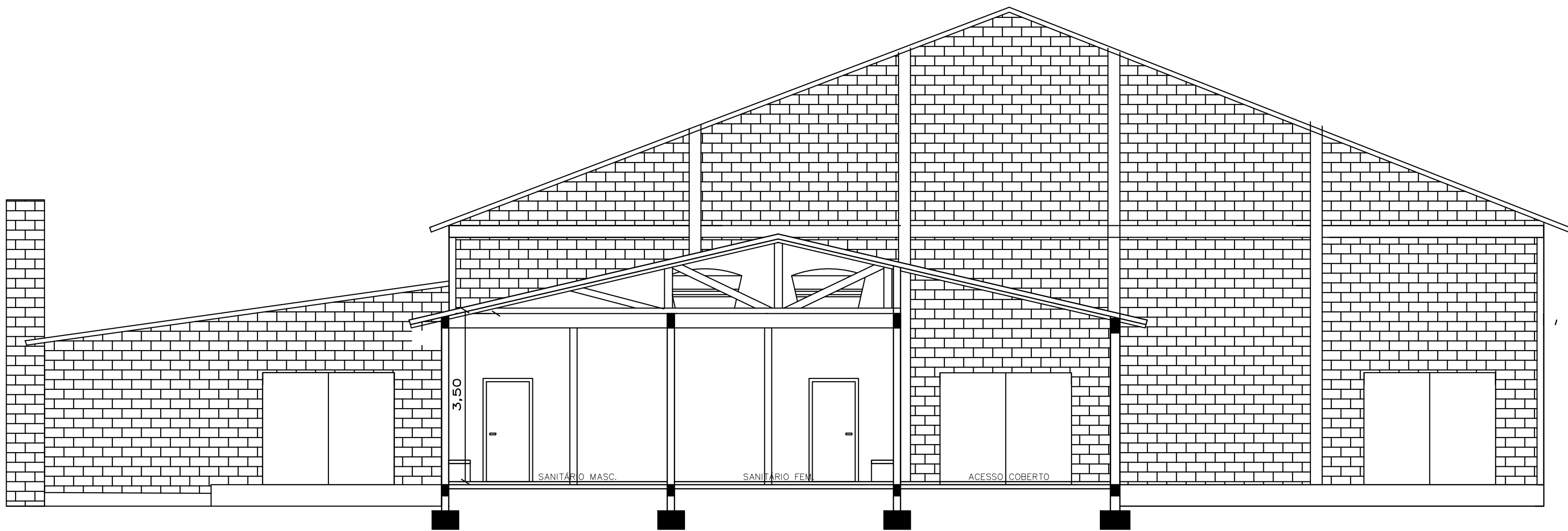
CORTE A—A
