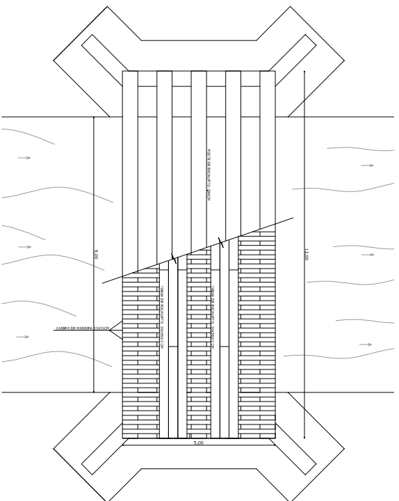
PLANTA BAIXA 1/50
