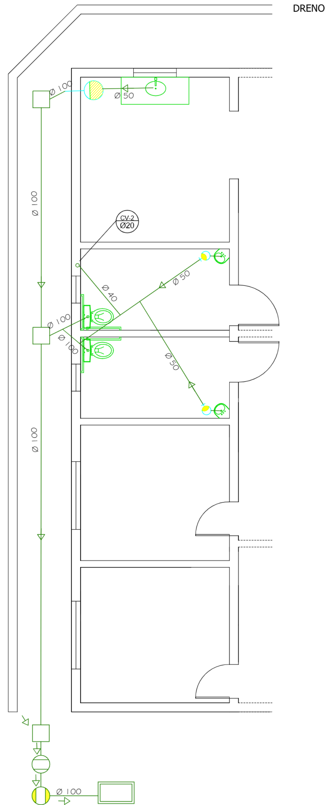
Planta Baixa Instalações de Esgoto Escala 1:50
