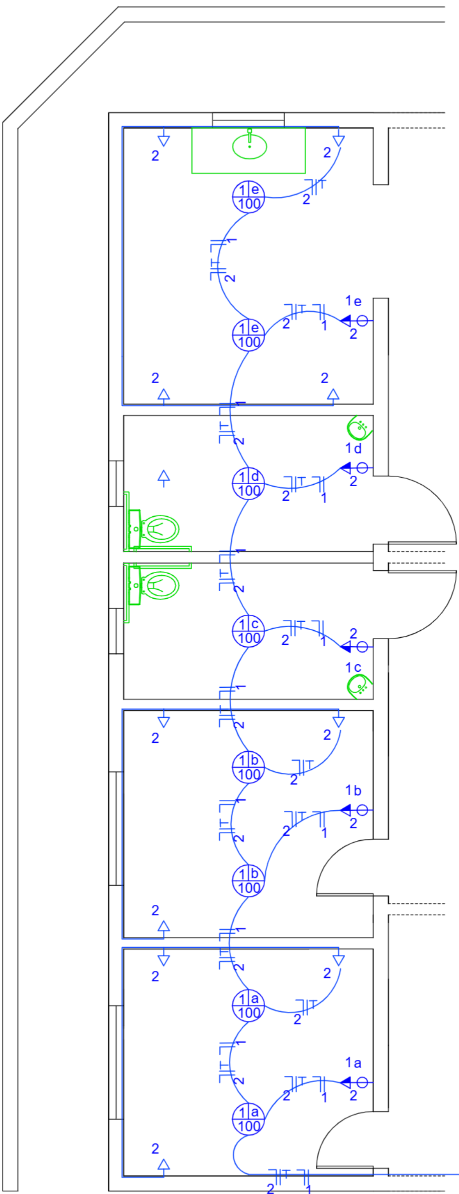
Planta Baixa Instalações Elétricas Escala 1:50
