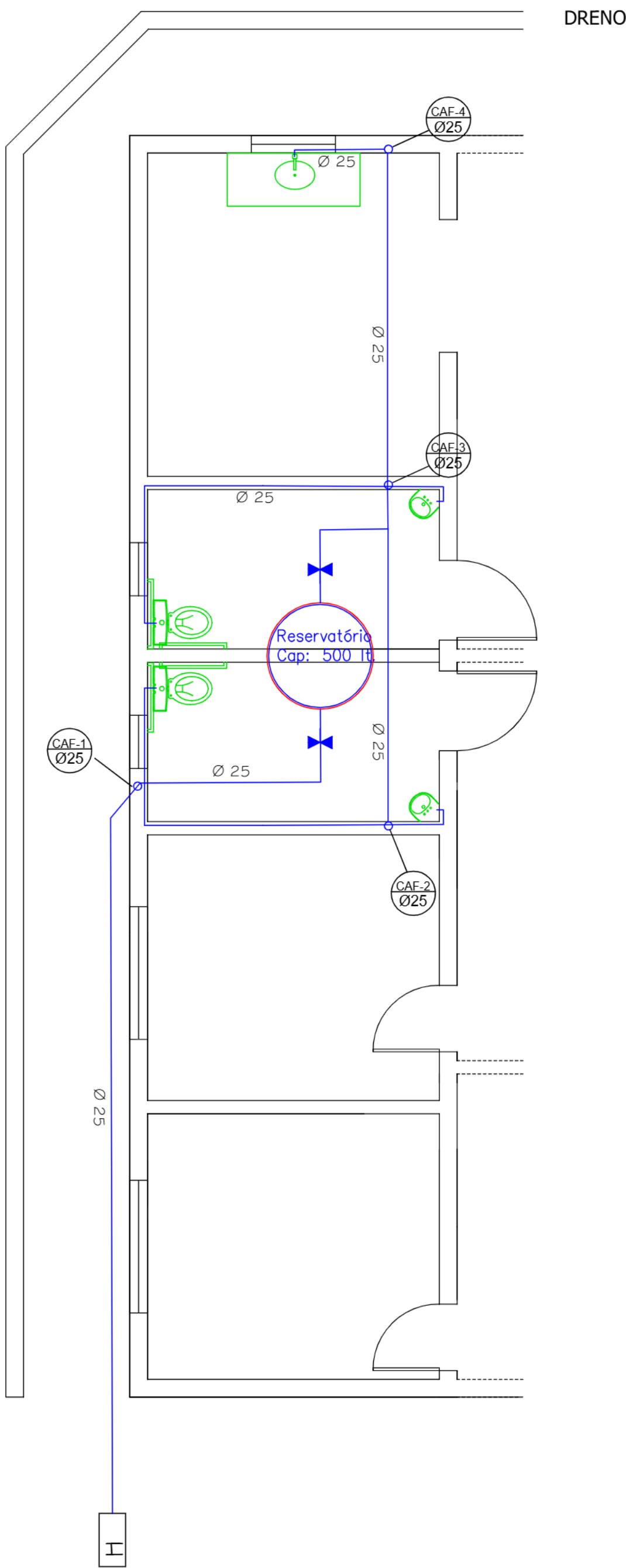
Planta Baixa Instalações de Água fria Escala 1:50
