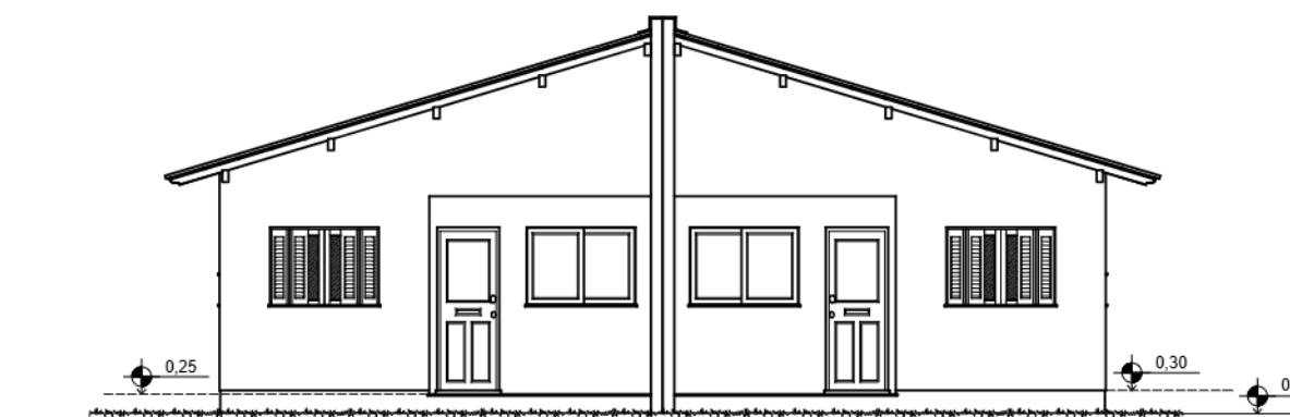
1 Elevação Frontal 1:100
