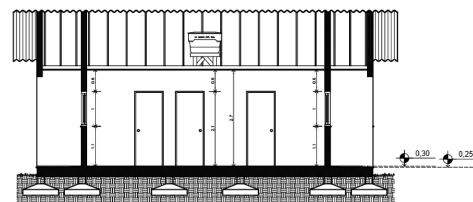
CD Corte 1:100
