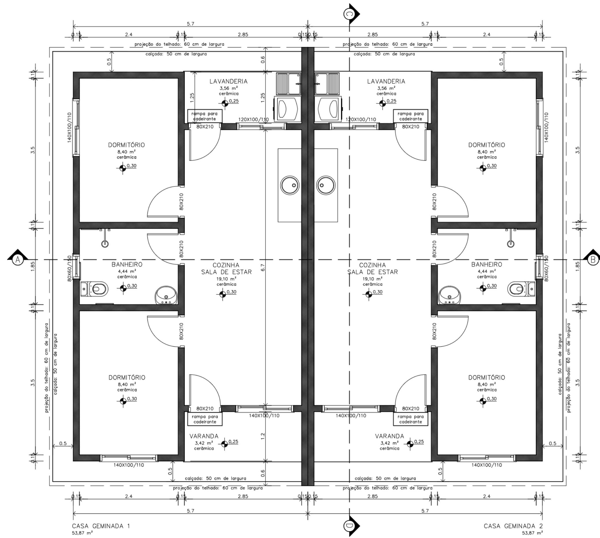
Planta Térreo 1:50
