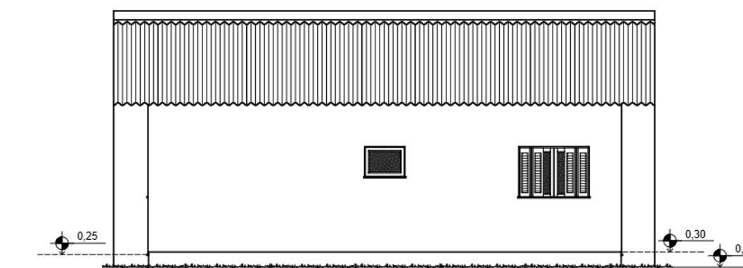
2 Lateral Direita 1:100
