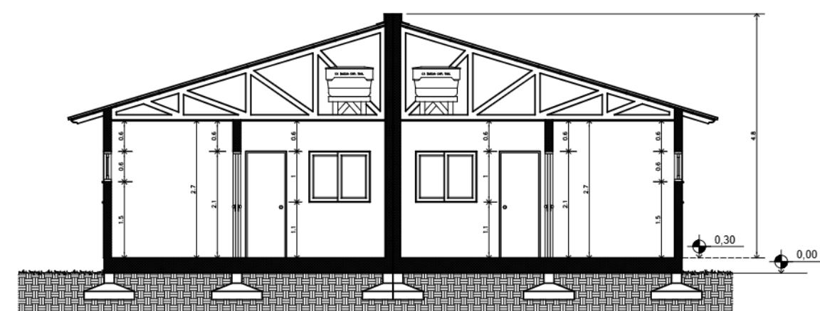
AB Corte 1:100
