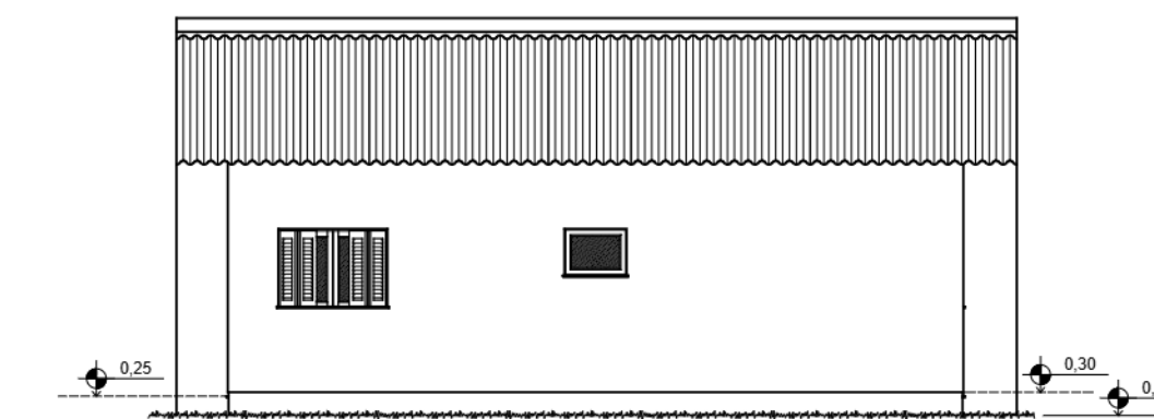
4 Lateral Esquerda 1:100
