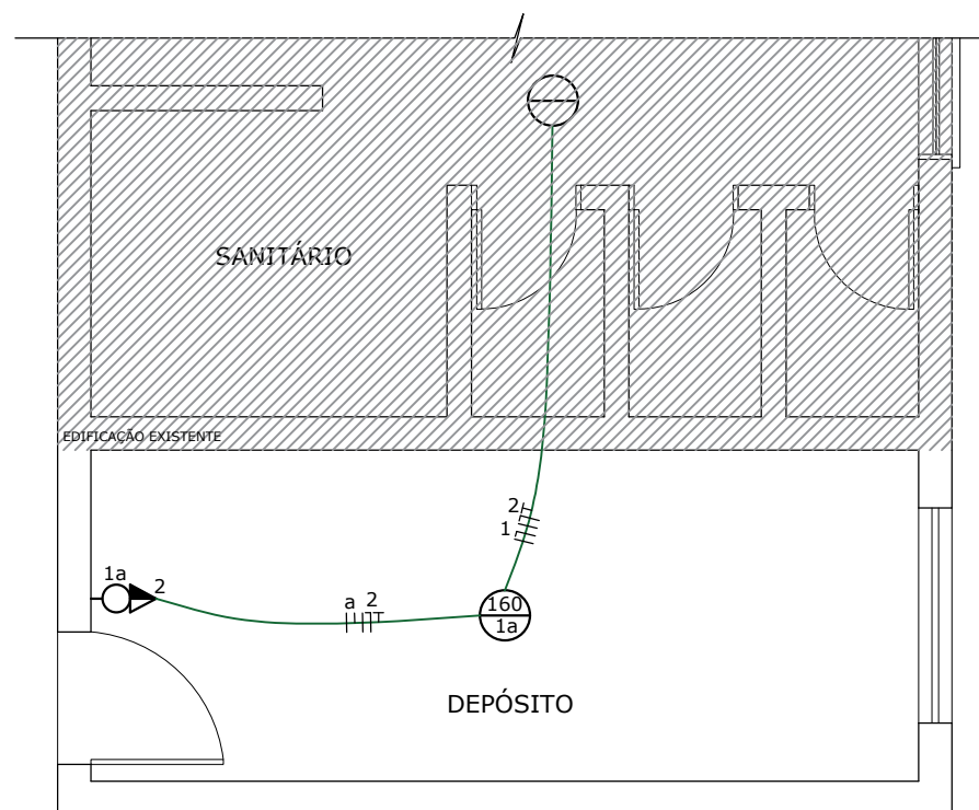
ESQUEMA DE INSTALAÇÃO ELÉTRICA esc. 1/50
