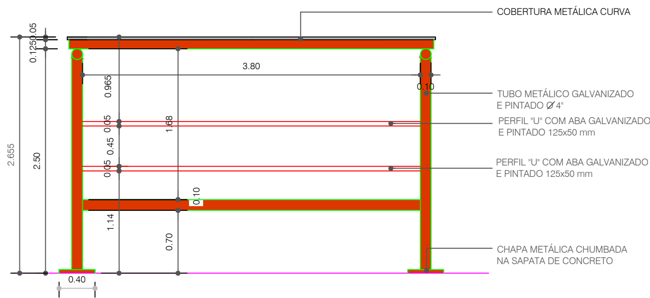
VISTA FRONTAL (SEM TESTEIRA) ESC. 1/50
