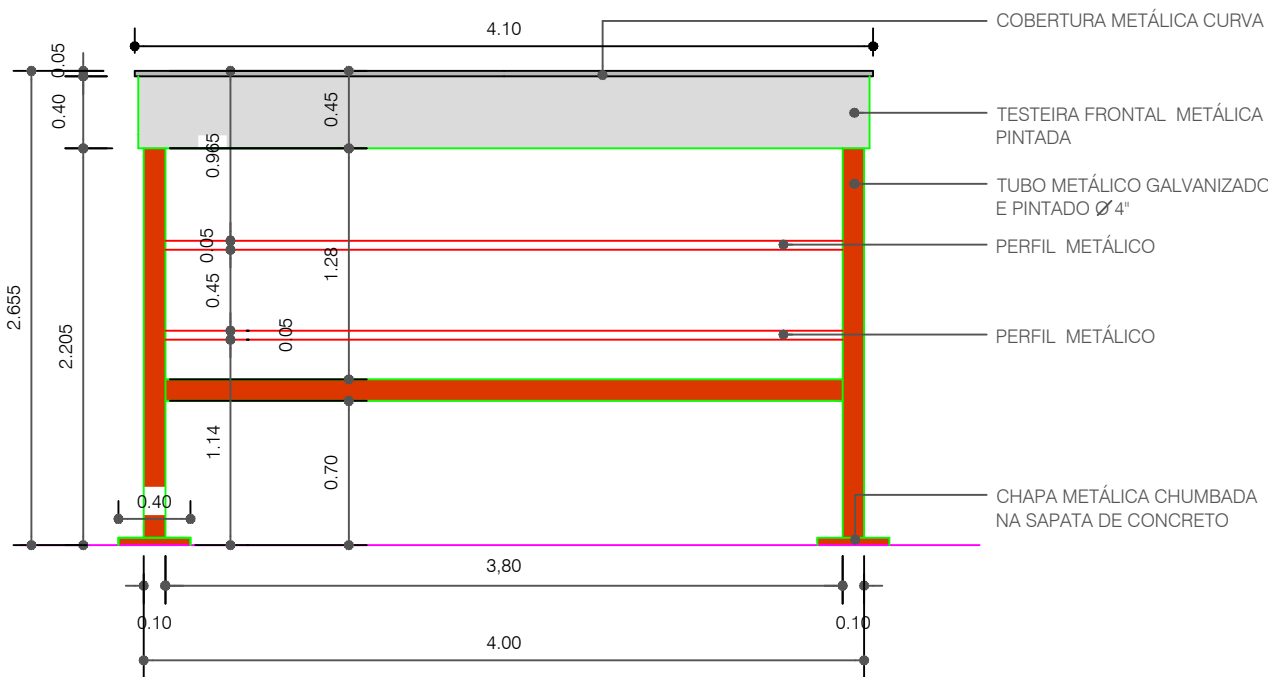
VISTA FRONTAL (COM TESTEIRA) ESC. 1/50
