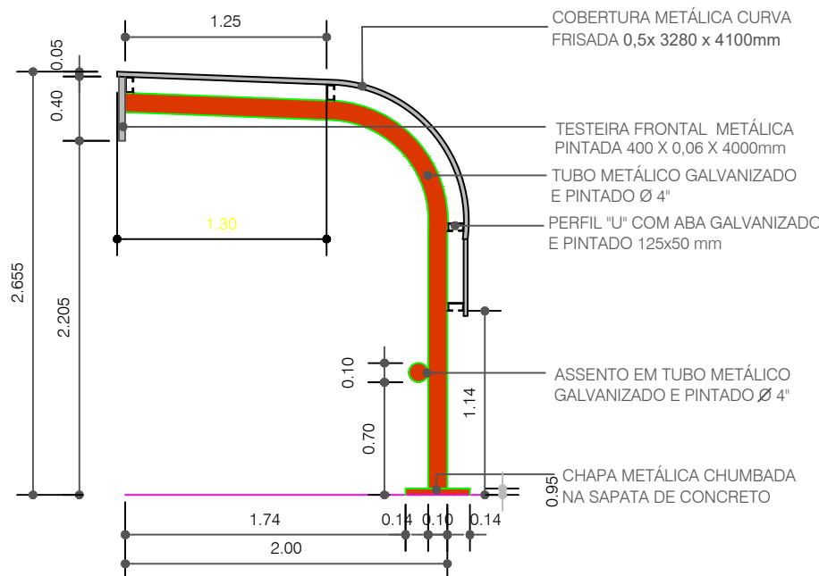
VISTA LATERAL ESC. 1/50
