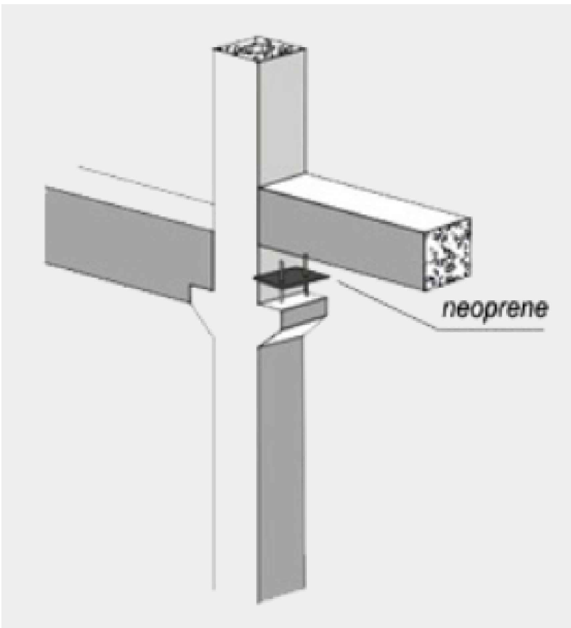
LIGAÇÃO VIGA E CONSOLO DE PILAR
