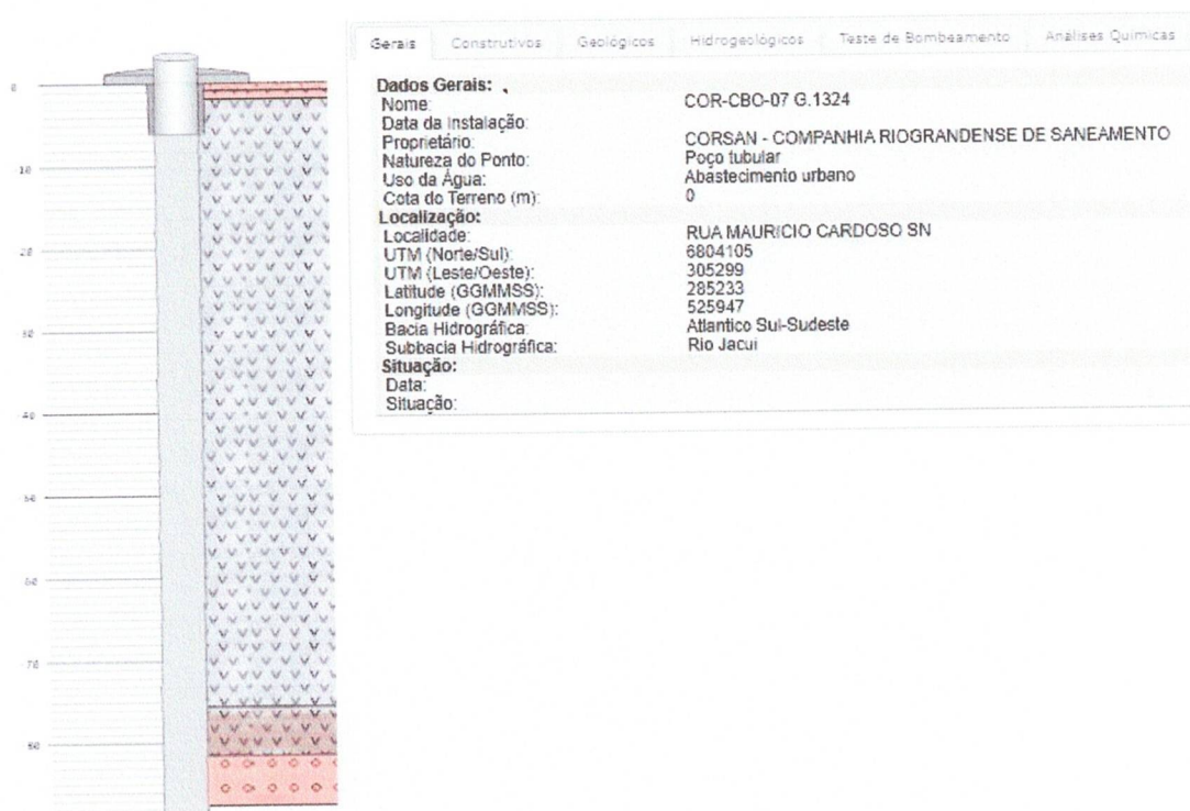
Figura 11: Perfil Geológico do Poço 1. Fonte: SIAGAS (2025).
