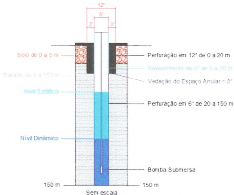
Figura 13: Perfil Geológico do Poço. Fonte: Autor (2025).
