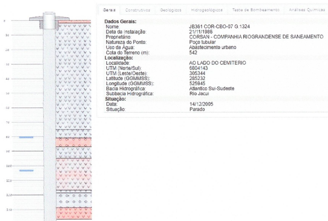
Figura 12: Perfil Geológico do Poço 2. Fonte: SIAGAS (2025).
