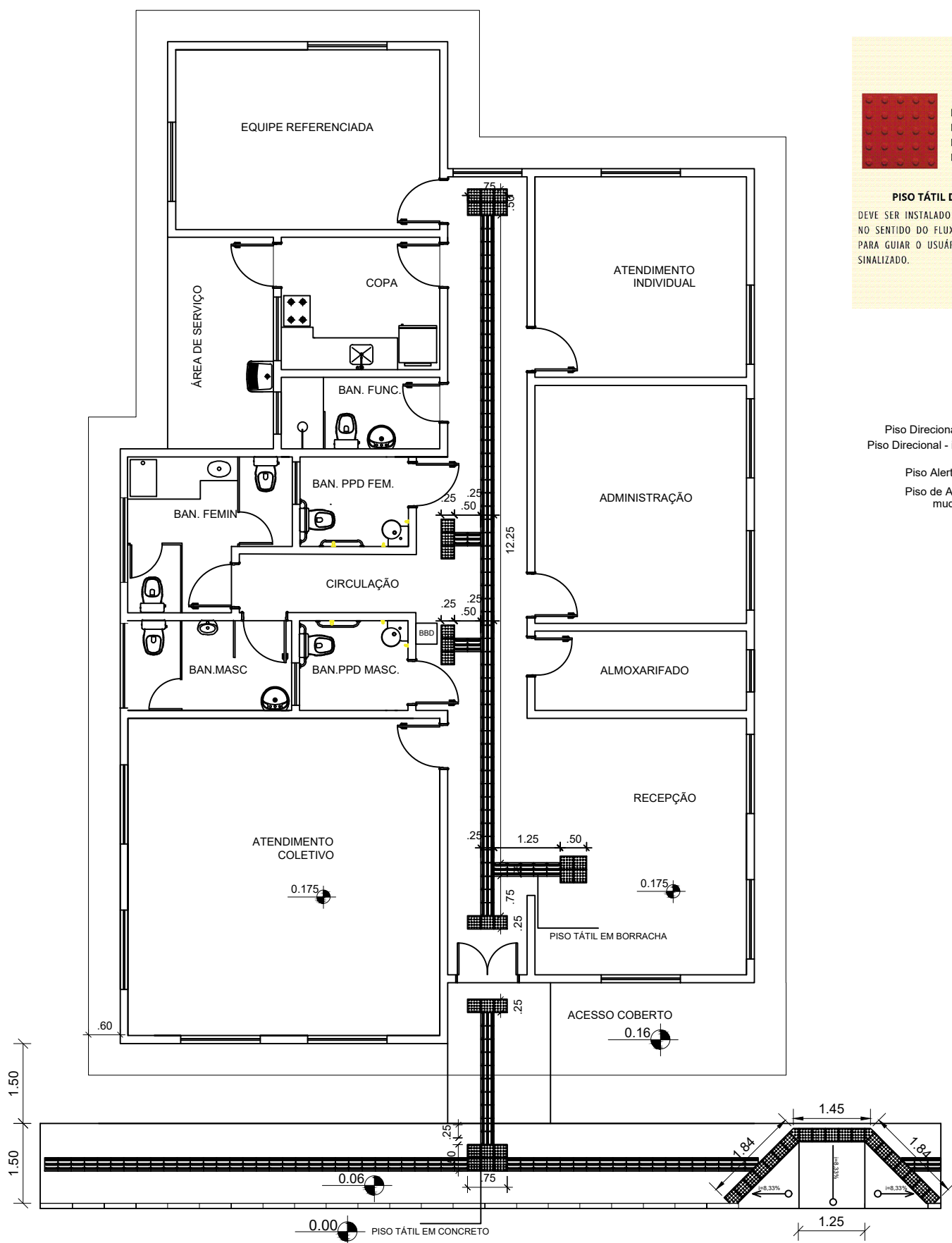
ACESSIBILIDADE ESCALA 1:100
