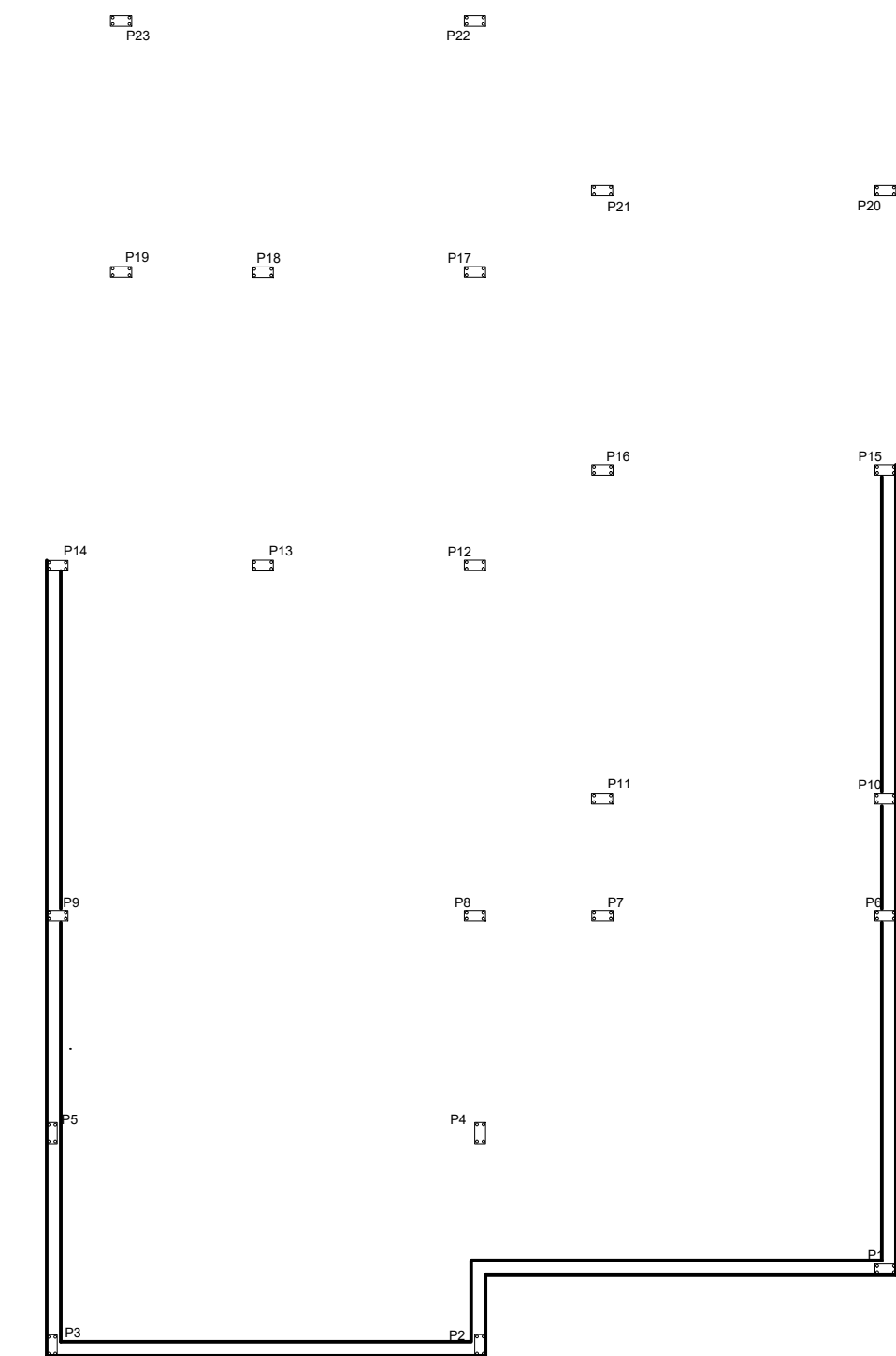
01 PLANTA VIGAS BALDRAME ESCALA: 1/100
