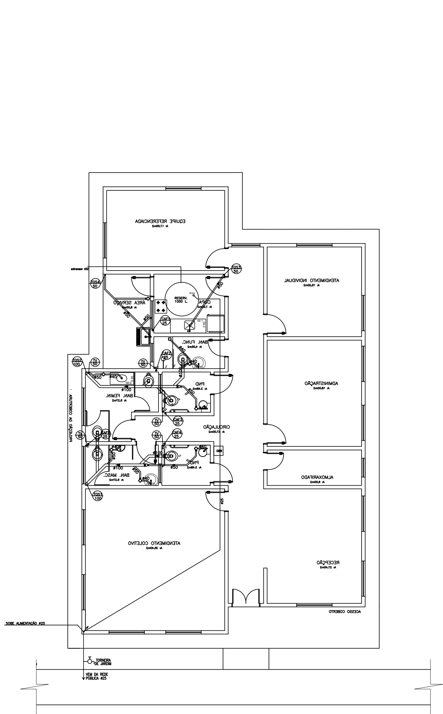
INSTALAÇÕES HIDROSSANITÁRIAS ESCALA 1:100
