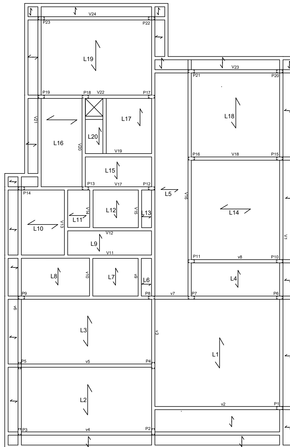
03 PLANTA VIGAS COBERTURA ESCALA: 1/100
