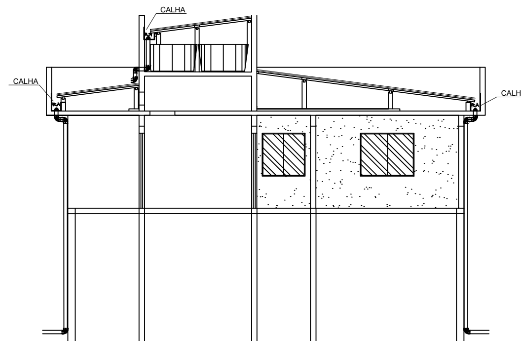
CORTE - DETALHAMENTOS PLUVIAL ESCALA 1:100
