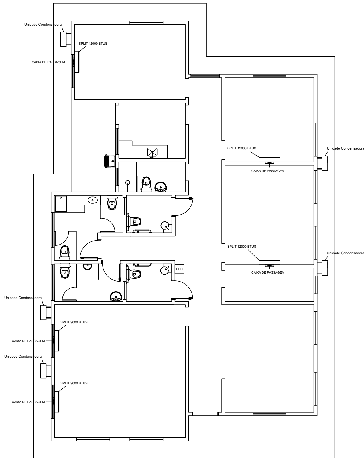
AR-CONDICIONADO ESCALA 1:100
