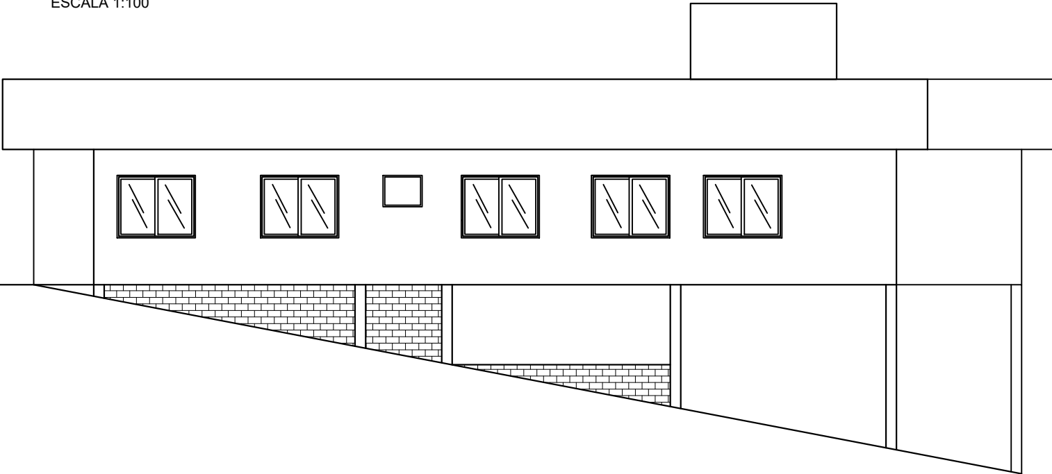
FACHADA LATERAL DIREITA ESCALA 1:100
