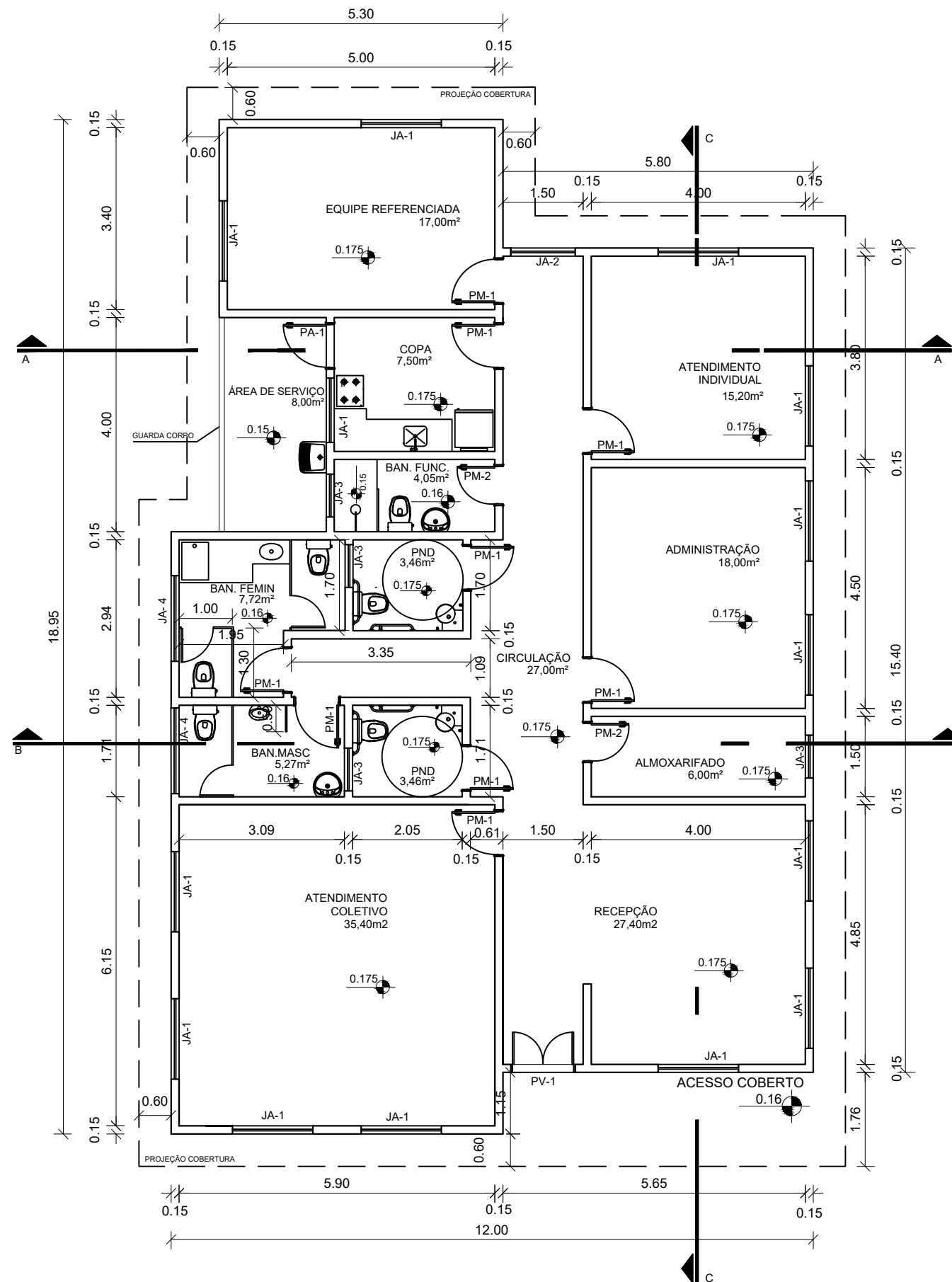
PLANTA BAIXA ESCALA 1:100
