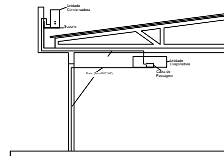
DETALHAMENTO AR-CONDICIONADO
