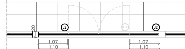
Janela J2 Dimensão: 110x213cm Peitoril: 5cm Quantidade: 2 unidades
