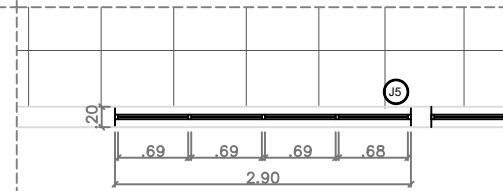
Janela J5 Dimensão: 290x100cm Peitoril: 155cm Quantidade: 4 unidades
