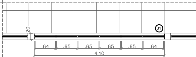
Janela J1 Dimensão: 410x100cm Peitoril: 155cm Quantidade: 3 unidades
