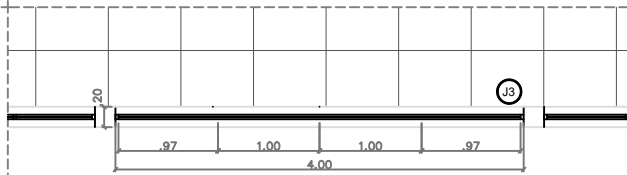
Janela J3 Dimensão: 400x37cm Peitoril: 215cm Quantidade: 1 unidade
