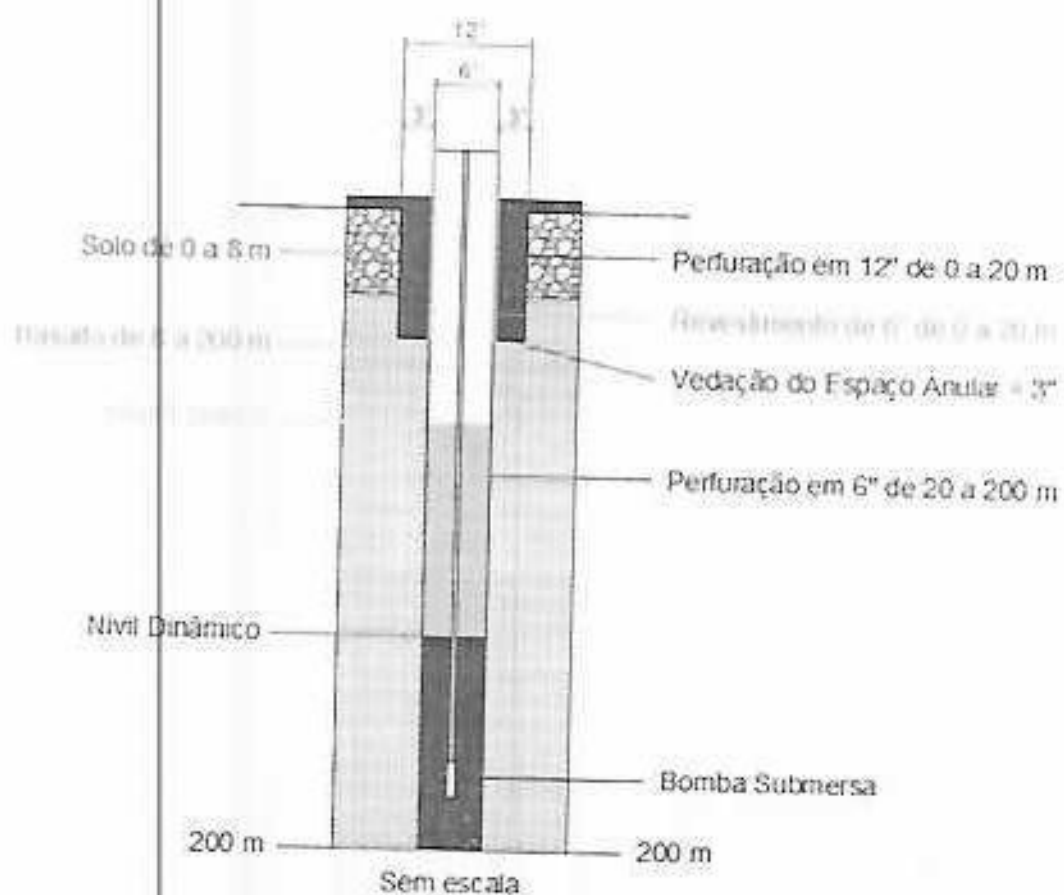
Perfil Geológico e Construtivo
