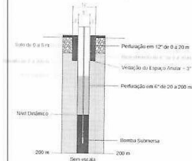
Figura 12: Perfil Geológico e Construtivo do Poço. Fonte: Autor (2026).
