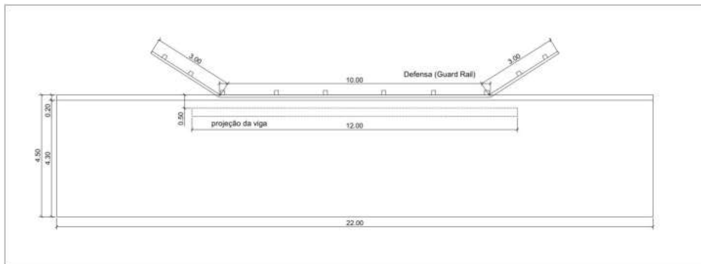
VISTA EM PLANTA
