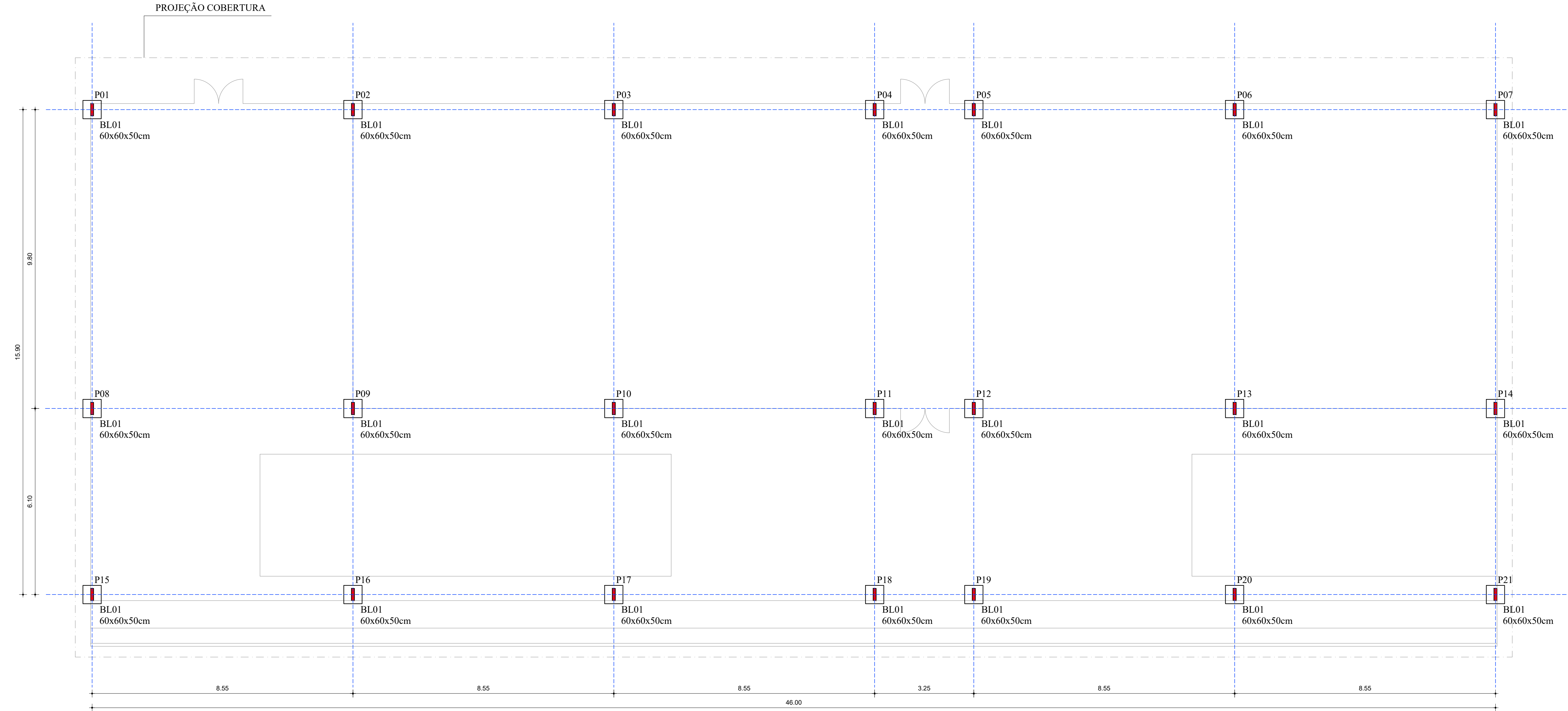
01 1/75 LOCAÇÃO DOS EIXOS DE PILARES E FUNDAÇÕES
