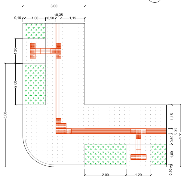
DETALHAMENTO ESQUINA
