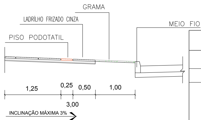
SEÇÃO TRANSVERSAL
