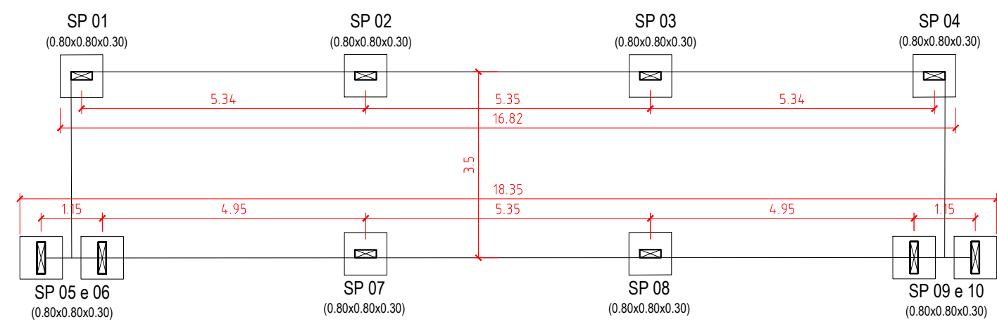
BLOCOS SAPATAS ESCALA: 1/100
