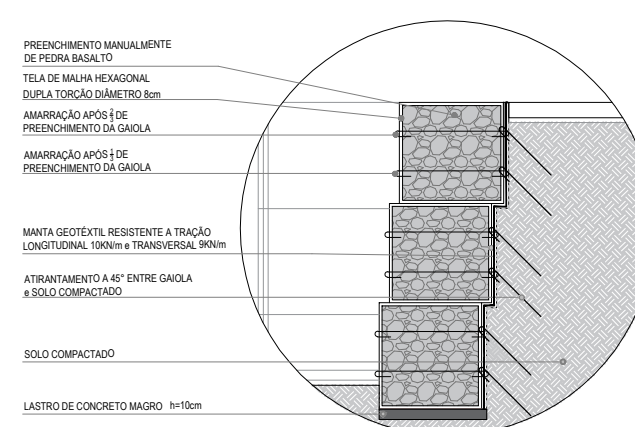
DETALHAMENTO MURO GABIÃO ESCALA: 1/75
