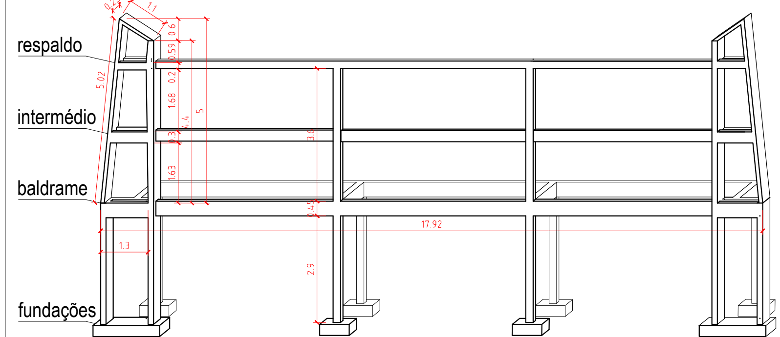
ESTRUTURAL MONUMENTO / MURAL ESCALA: 1/100
