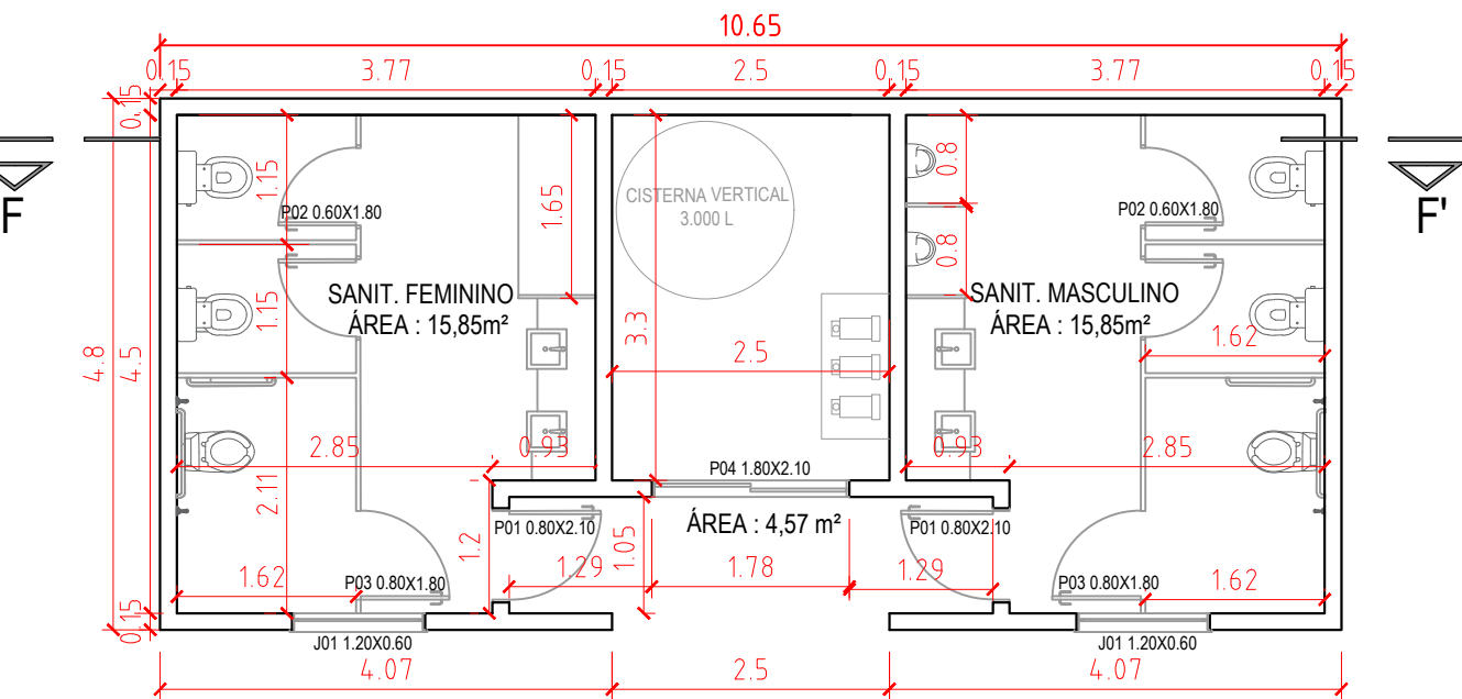
PLANTA BAIXA SANITÁRIOS E CASA DE MÁQUINAS ESCALA: 1/75
