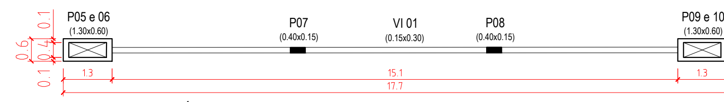
VIGA INTERMEDIÁRIA ESCALA: 1/100
