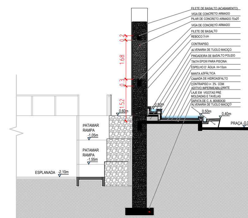
CORTE EE' ESCALA: 1/100
