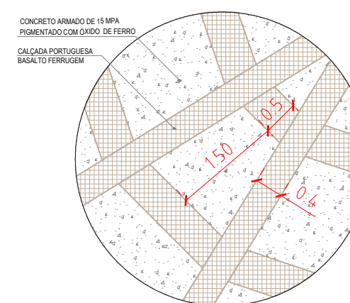
DETALHAMENTO PAVIMENTO ESCALA: 1/75
