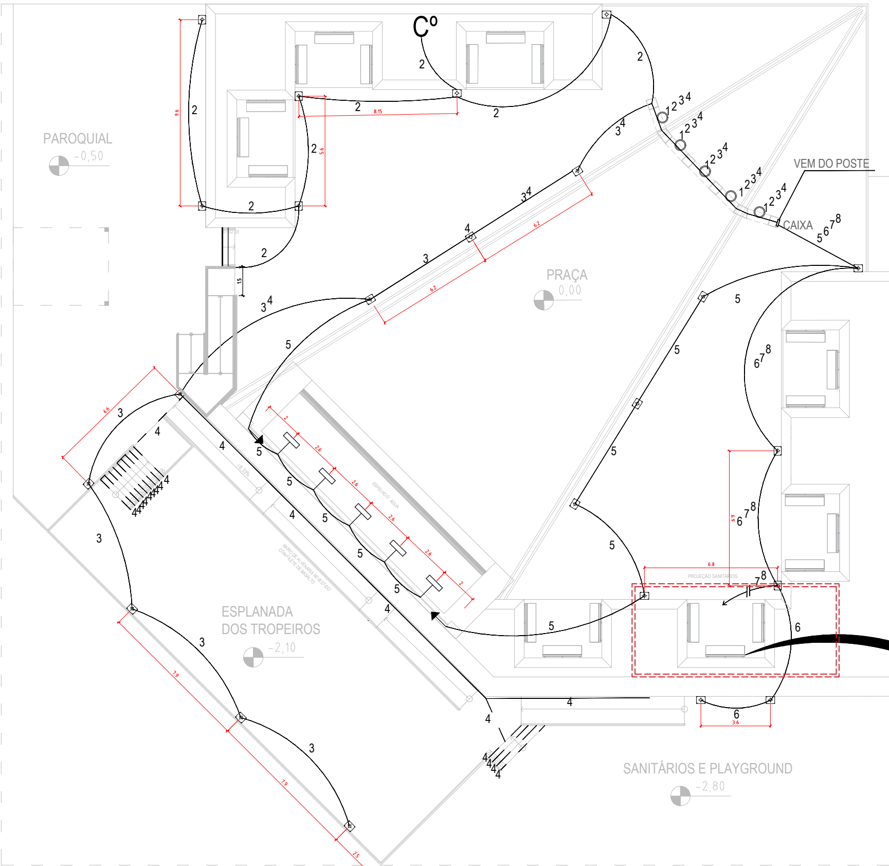
PLANTA BAIXA ELÉTRICA ESCALA: 1/200
