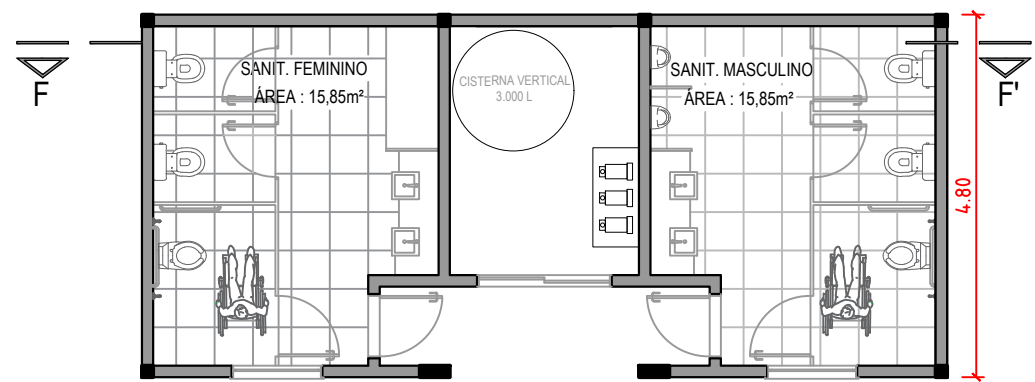
P.B. SANITÁRIOS E CASA DE MÁQUINAS ESCALA: 1/100
