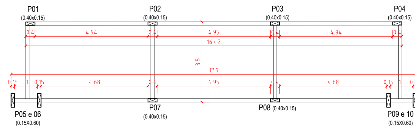
ARRANQUE DOS PILARES ESCALA: 1/100
