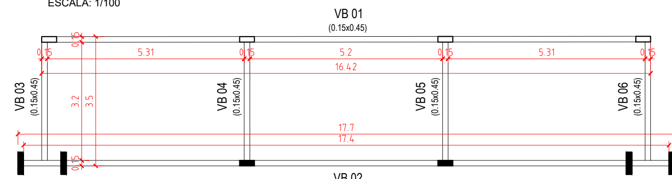
VIGA BALDRAME ESCALA: 1/100
