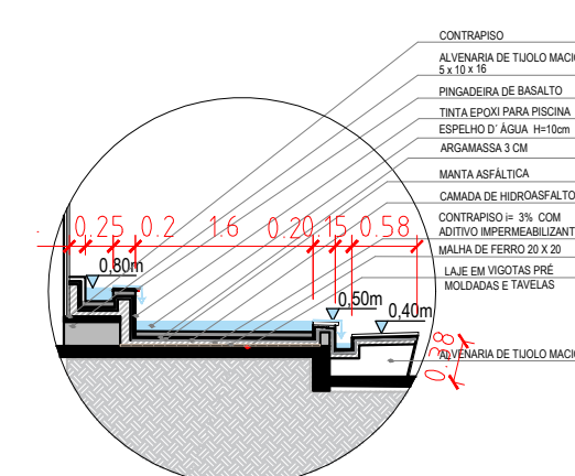
DETALHAMENTO ESPELHO D'ÁGUA MONUMENTO ESCALA: 1/75
