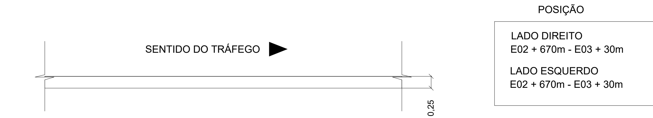
DETALHE DETALHE DE LINHA CONTÍNUA Tinta: HOT SPRAY Cor: BRANCA
