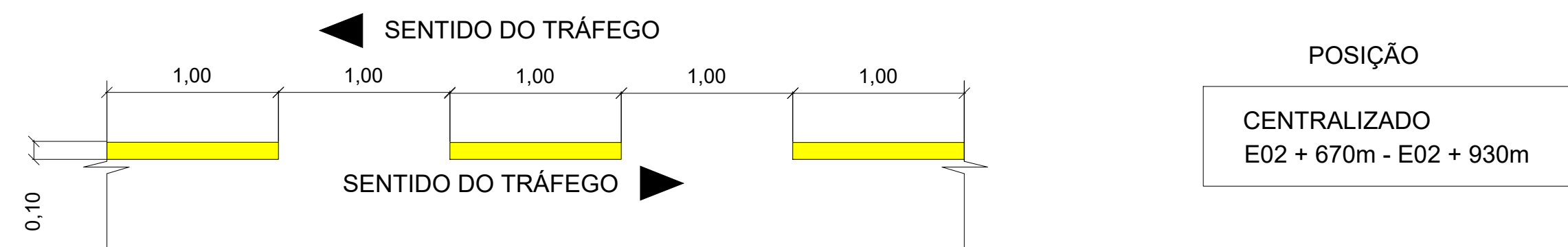
DETALHE DETALHE DE LINHA TRACEJADA Tinta: HOT SPRAY Cor: BRANCA
