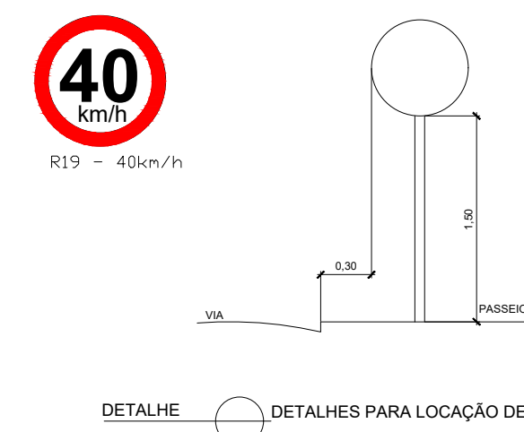
5 Sinalização Vertical Sem Escala
