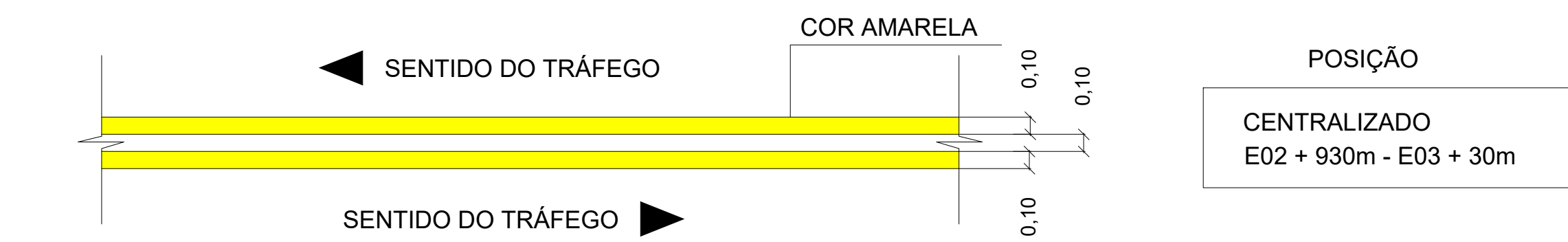
DETALHE DETALHE DE LINHA DUPLA AMARELA Tinta: HOT SPRAY Cor: AMARELA
