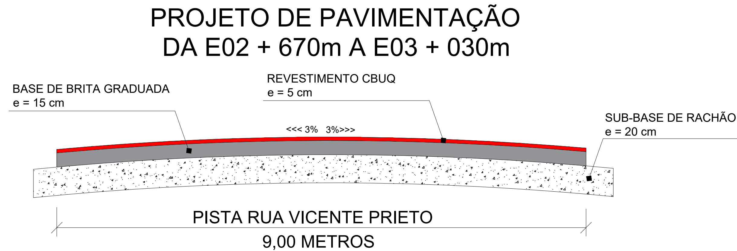
PERFIL TRANSVERSAL RUA VICENTE PRIETO
