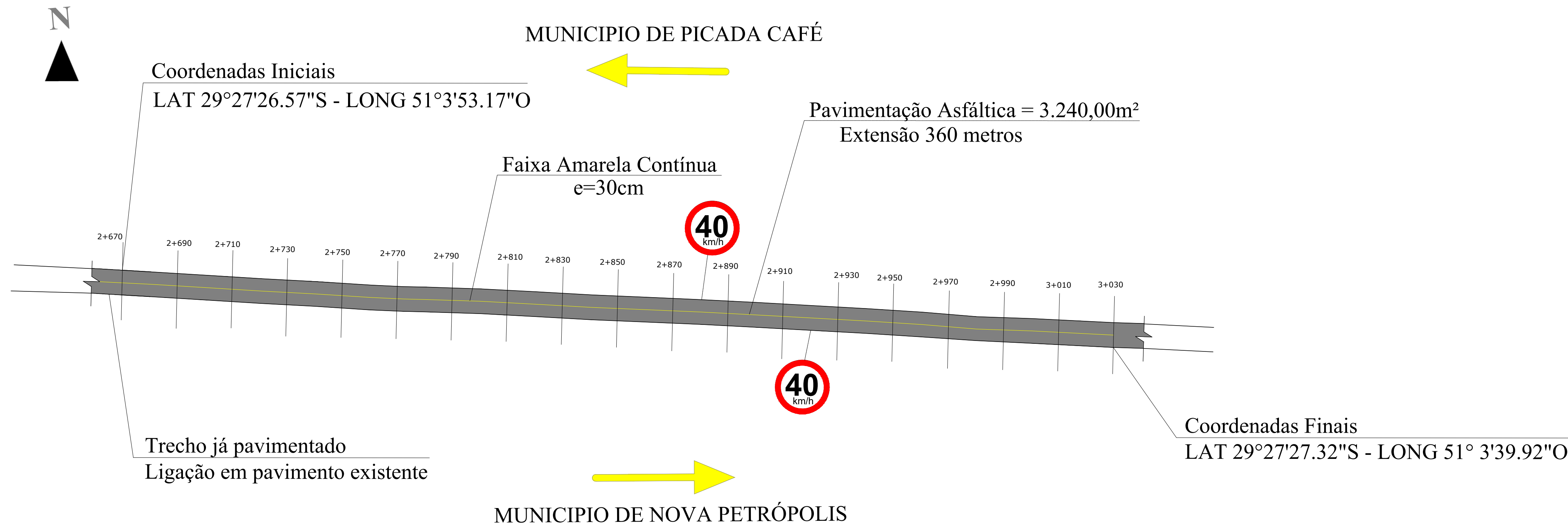
2 Planta Baixa 1:1000
