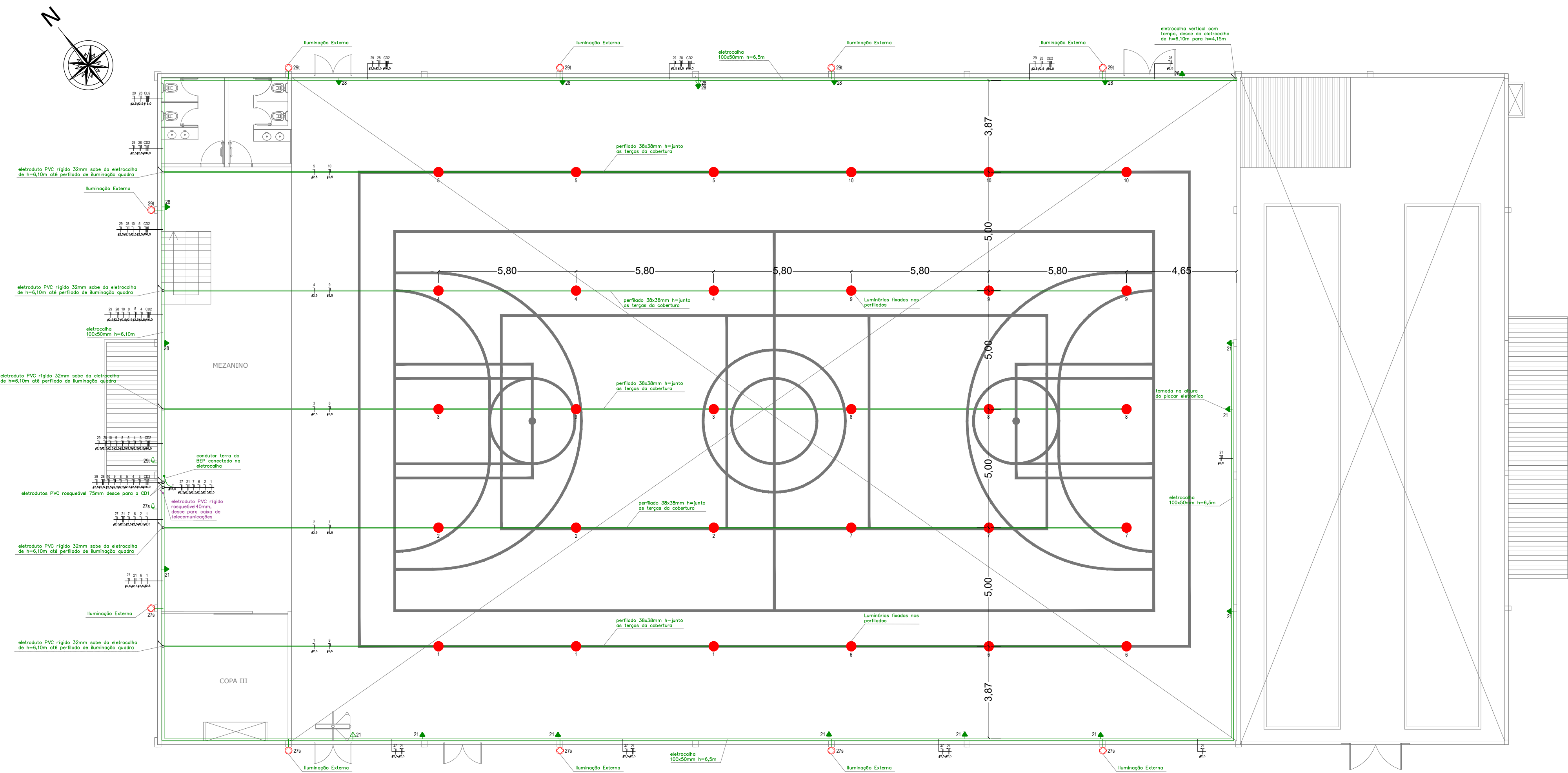
PLANTA MEZANINO - QUADRA DE ESPORTES NP ESCALA: 1/125
