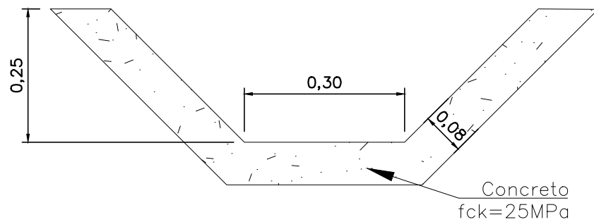
DR-3B-3 Corte Esc.: 1:10
