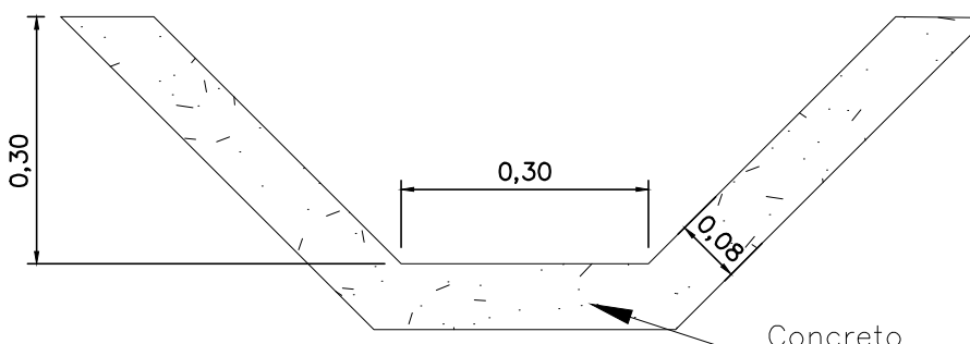
DR-3B-4 Corte Esc.: 1:10
