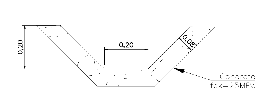
DR-3B-1 Corte Esc.: 1:10
