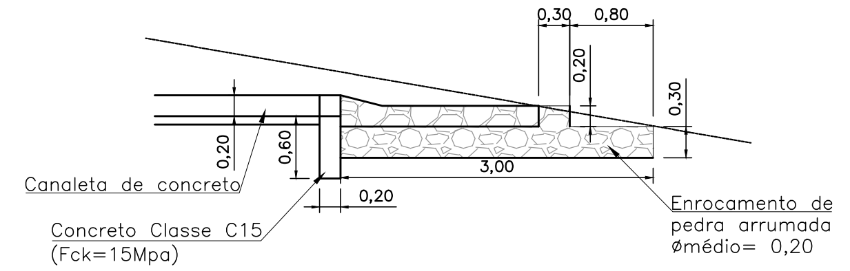
Dissipador de energia (DR-10A-2) Corte A ESC.: 1:50
