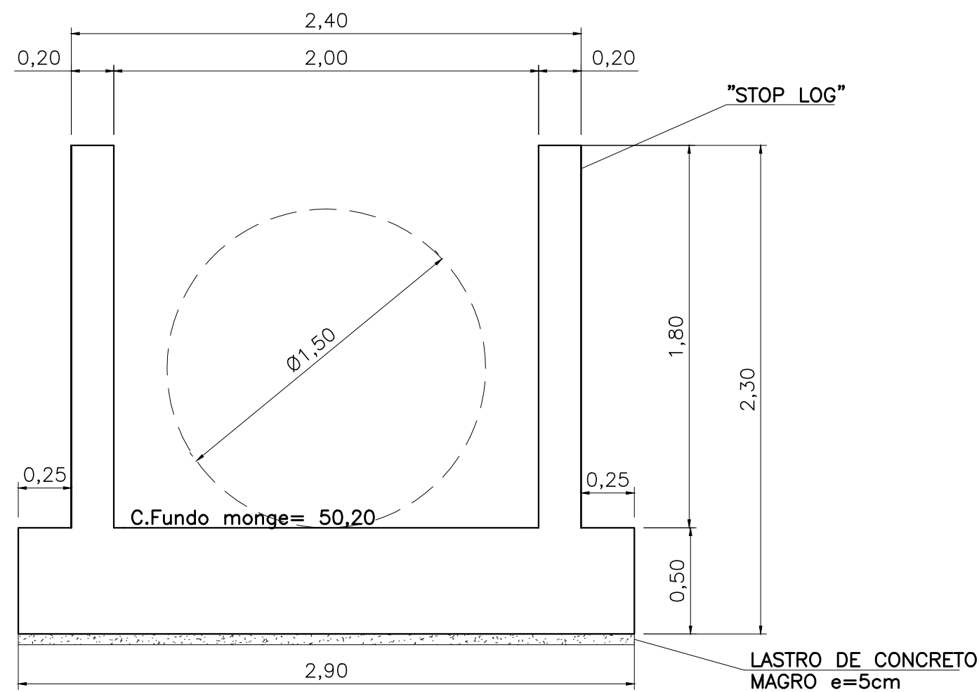
VERTEDOR MONGE E STOP-LOG CORTE B ESC.: 1:25
