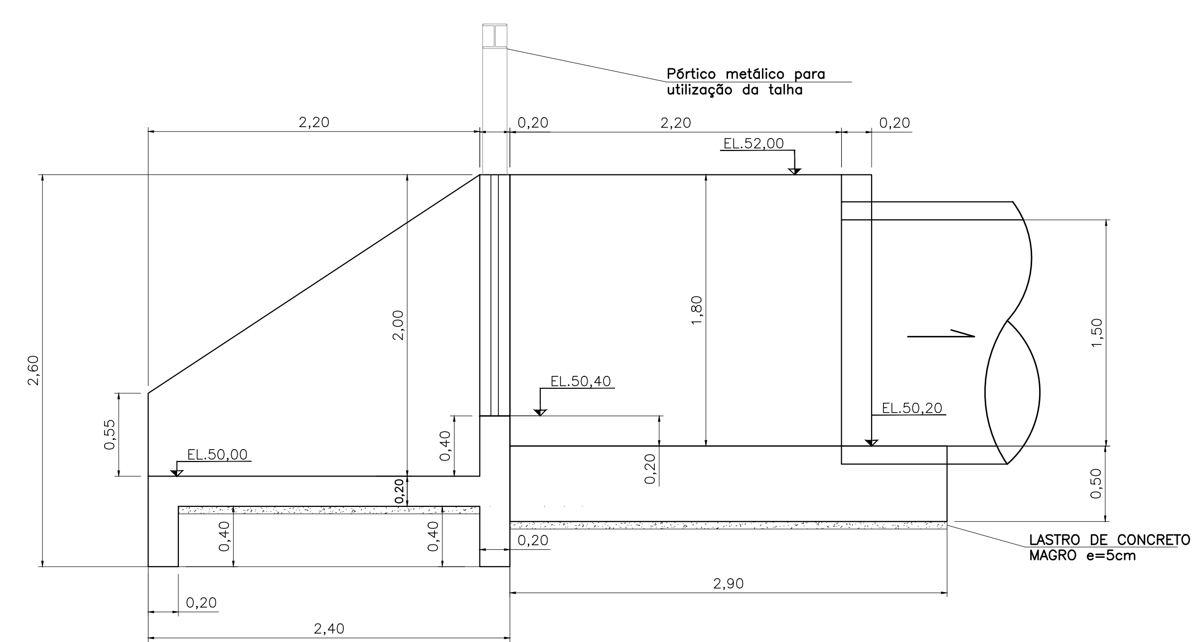
VERTEDOR MONGE E STOP-LOG CORTE A ESC.: 1:25
