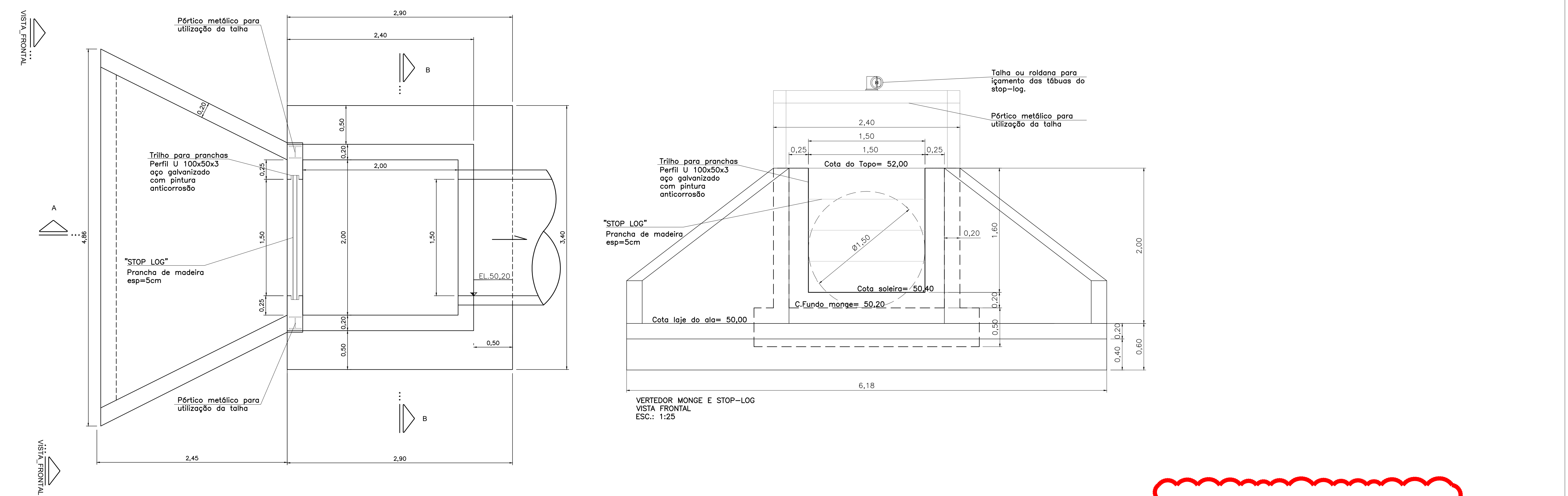
VERTEDOR MONGE E STOP-LOG PLANTA ESC.: 1:25
