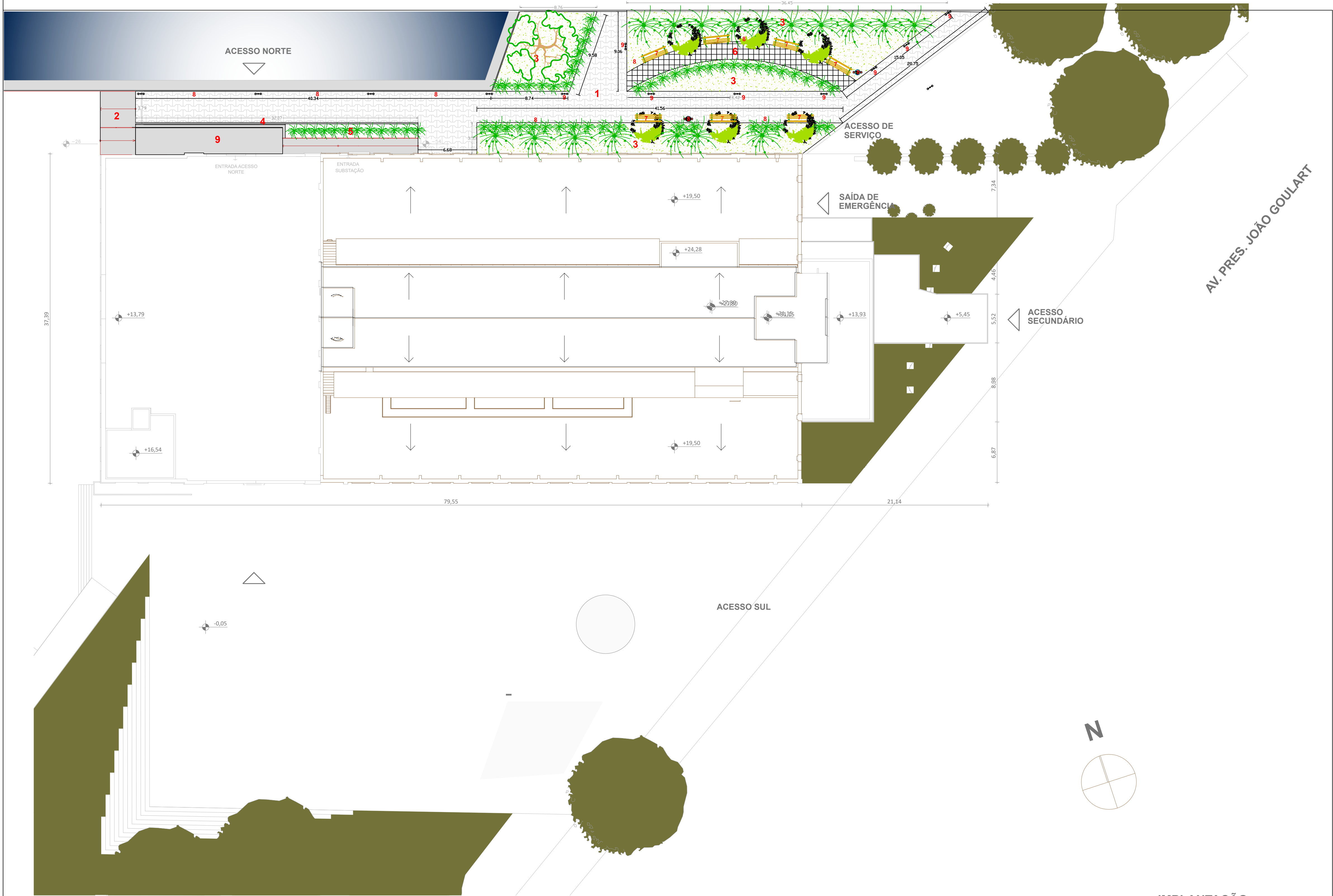
IMPLANTAÇÃO 1:150
