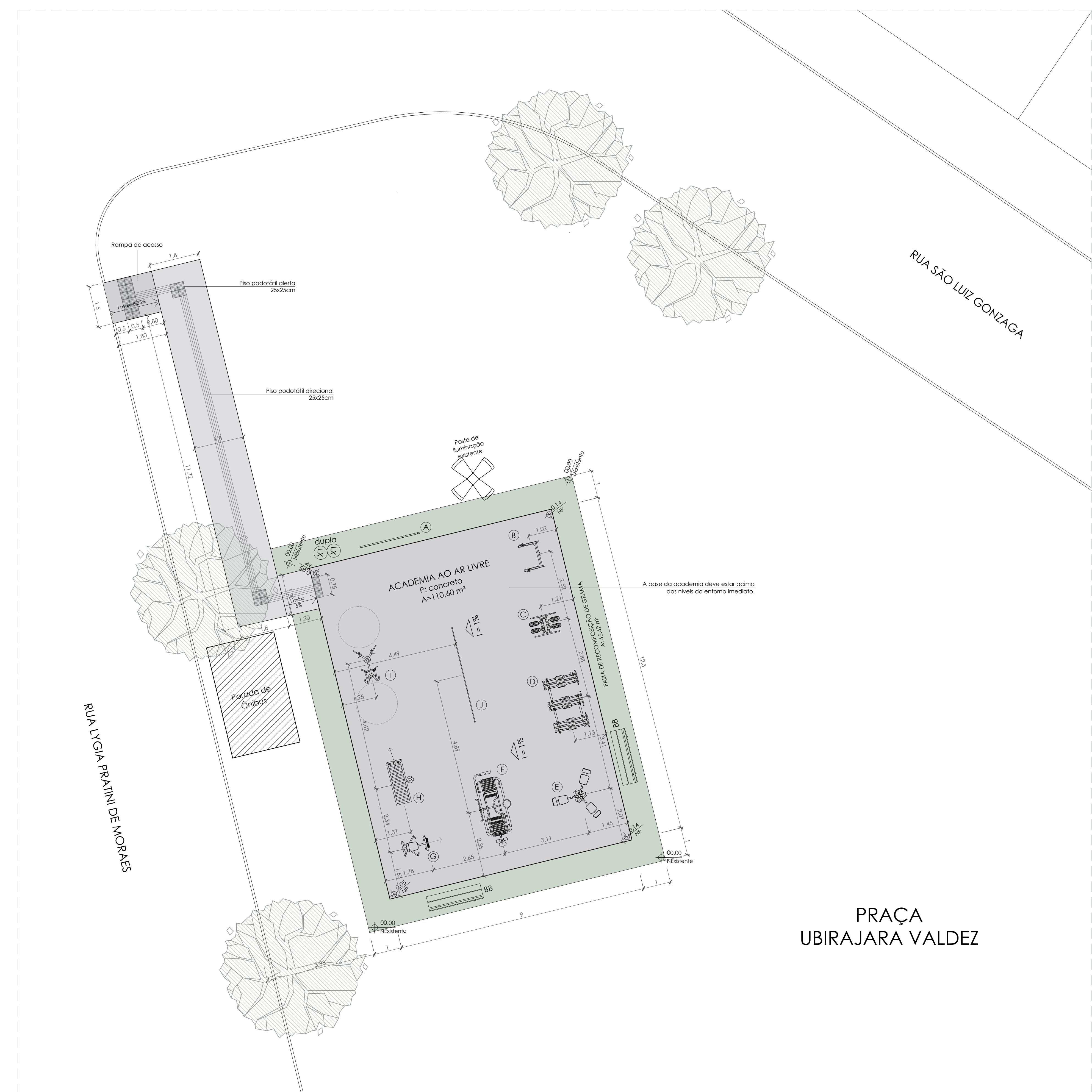
IMPLANTAÇÃO ESC. 1/100
