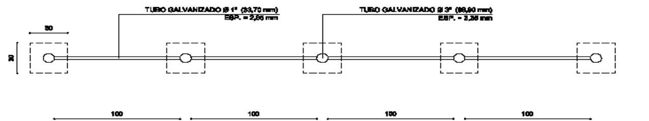
VISTA SUPERIOR
