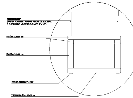
DETALHE 2 ESCALA 1:5
