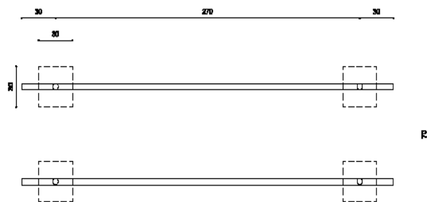
VISTA SUPERIOR
