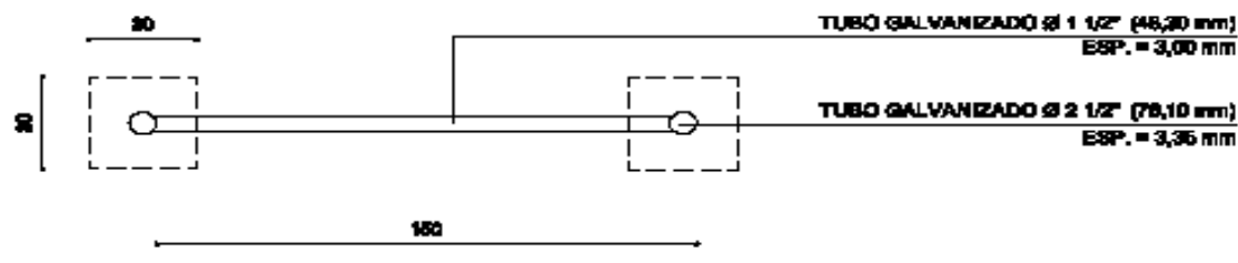
VISTA SUPERIOR
