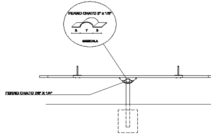
CORTE
