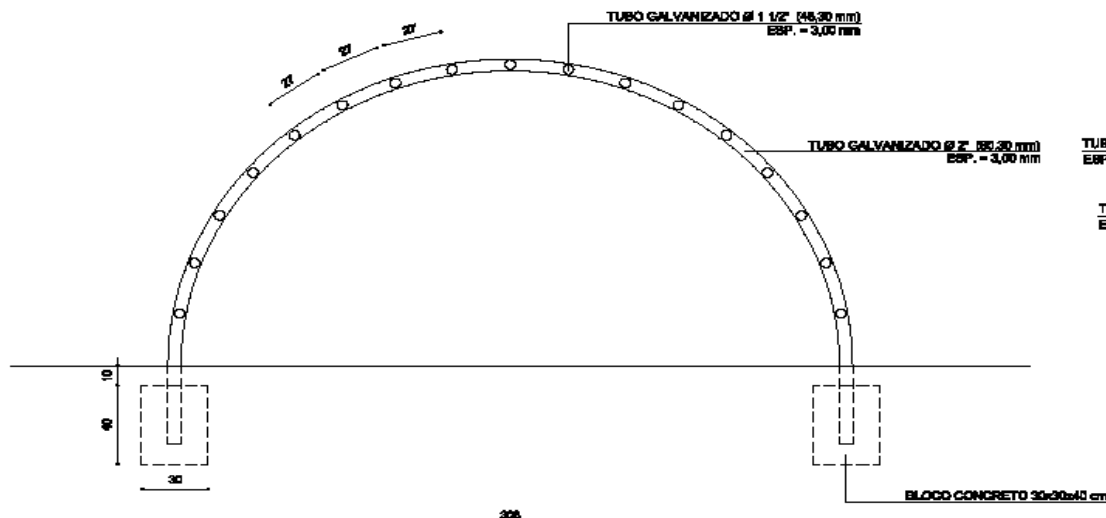
CORTE AA
