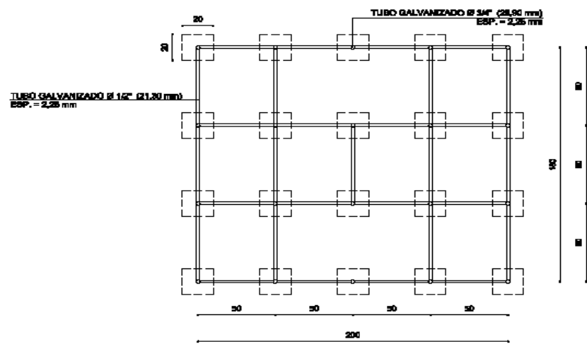
VISTA SUPERIOR
