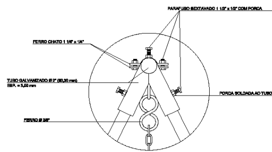
DETALHE 2 ESCALA 1:5
