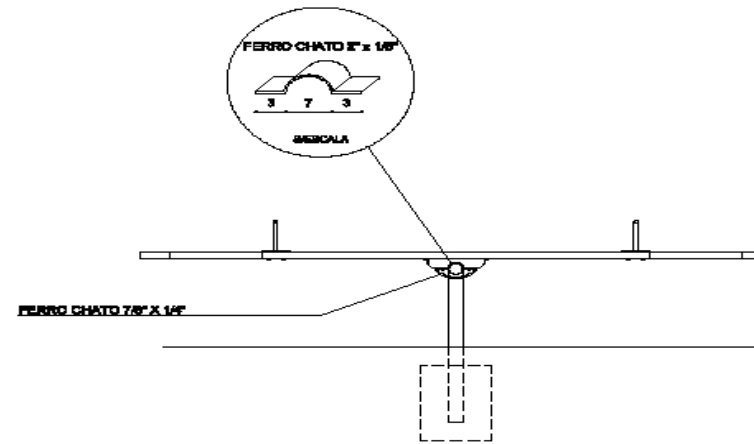
CORTE
