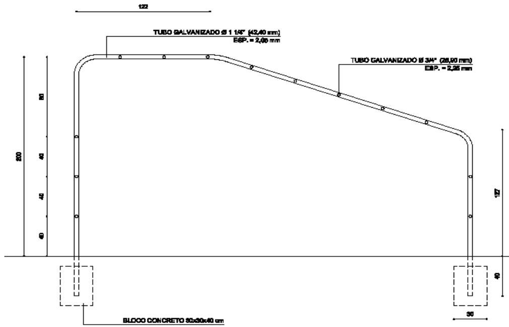
CORTE AA
