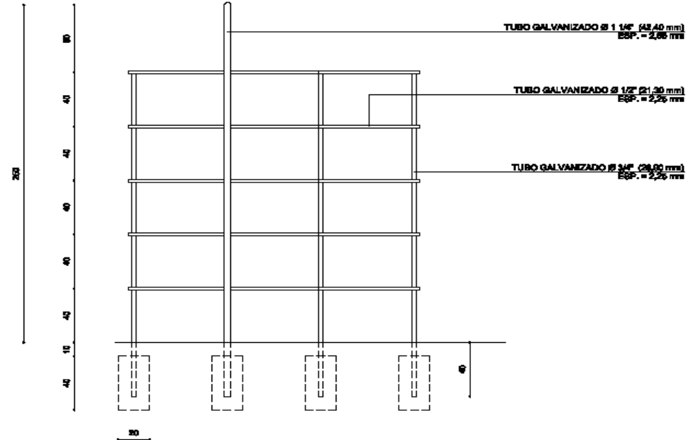
VISTA LATERAL
