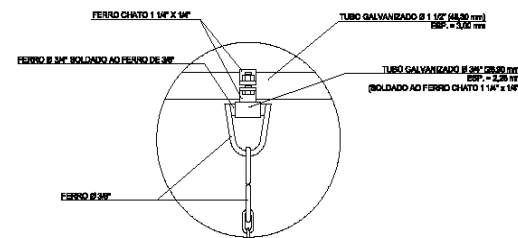
DETALHE 1 ESCALA 1:5
