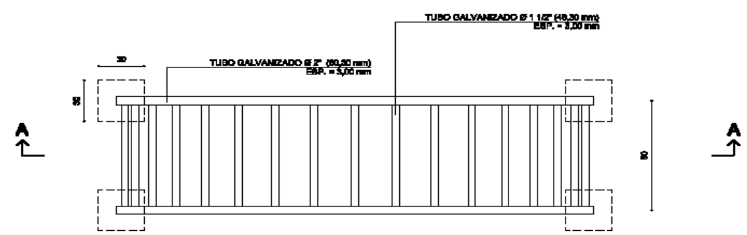
VISTA SUPERIOR
