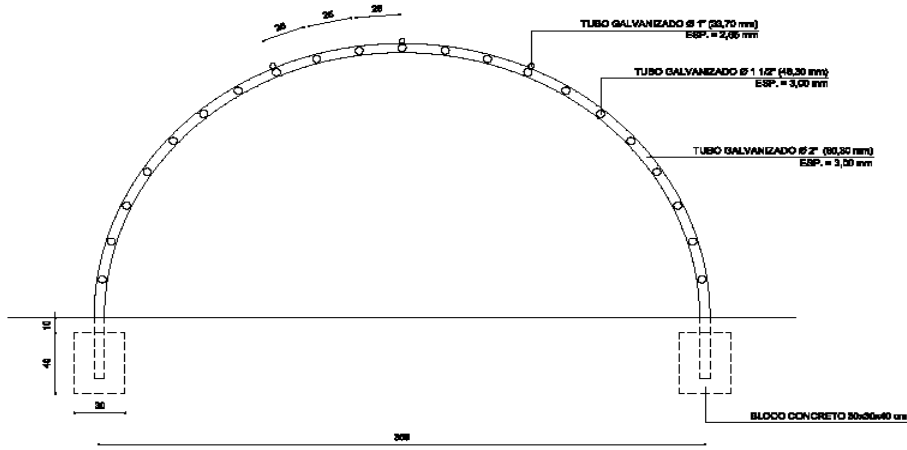
CORTE AA
