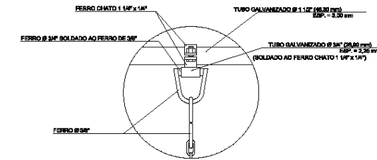
DETALHE 3 ESCALA 1:5
