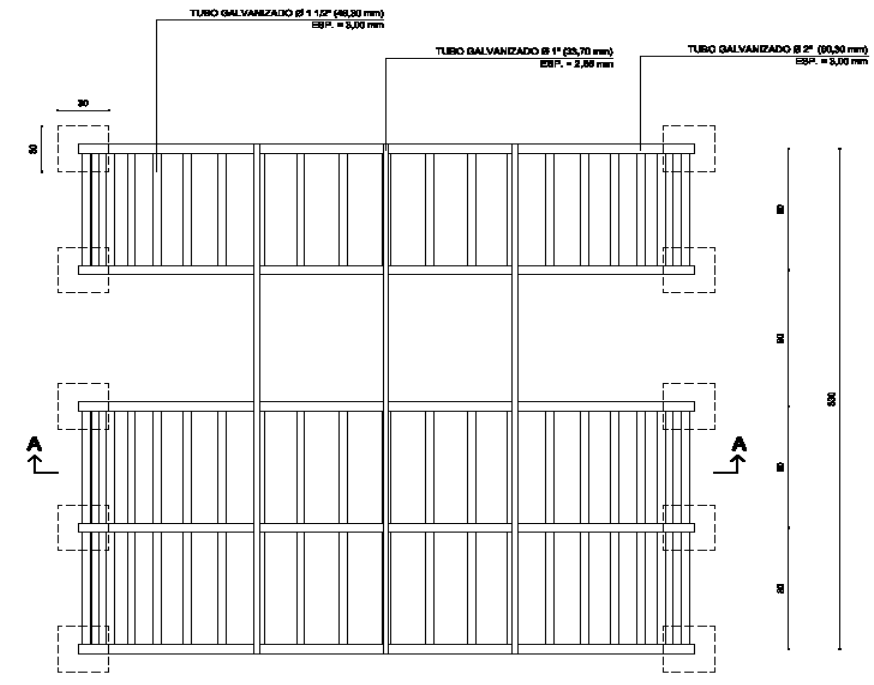
VISTA SUPERIOR
