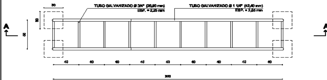
VISTA SUPERIOR
