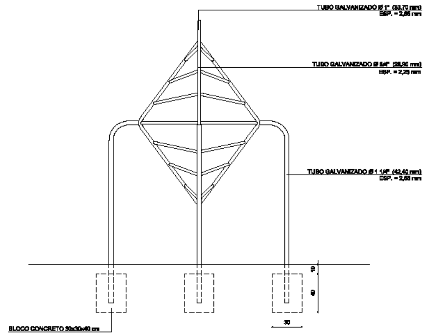
VISTA LATERAL
