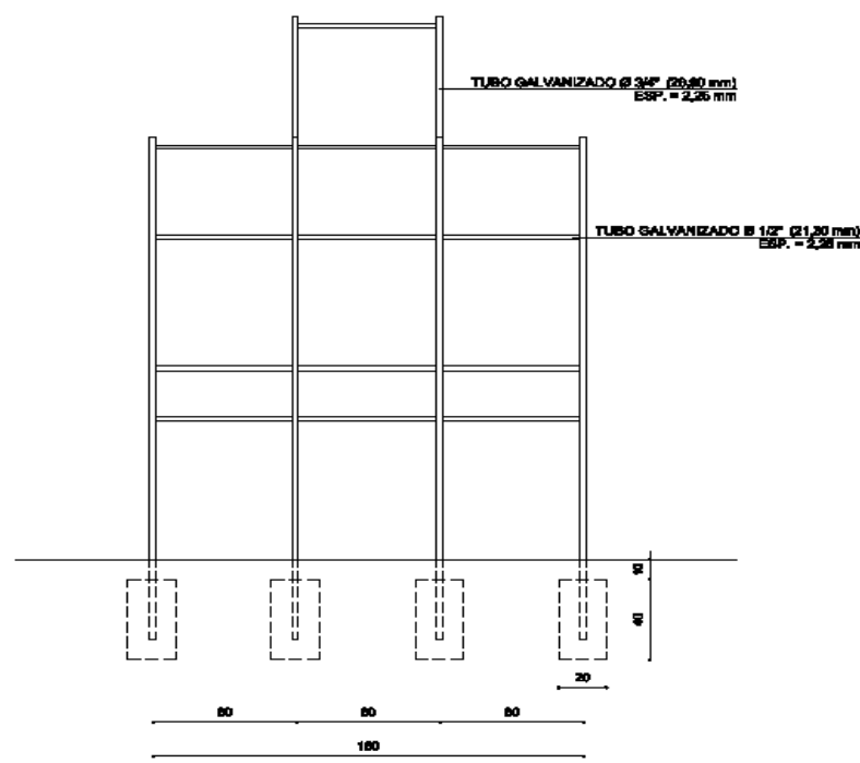
VISTA LATERAL
