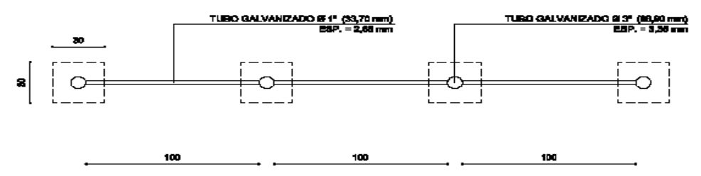
VISTA SUPERIOR
