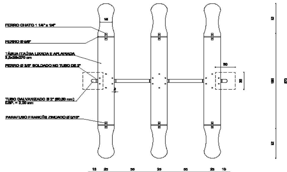
VISTA SUPERIOR
