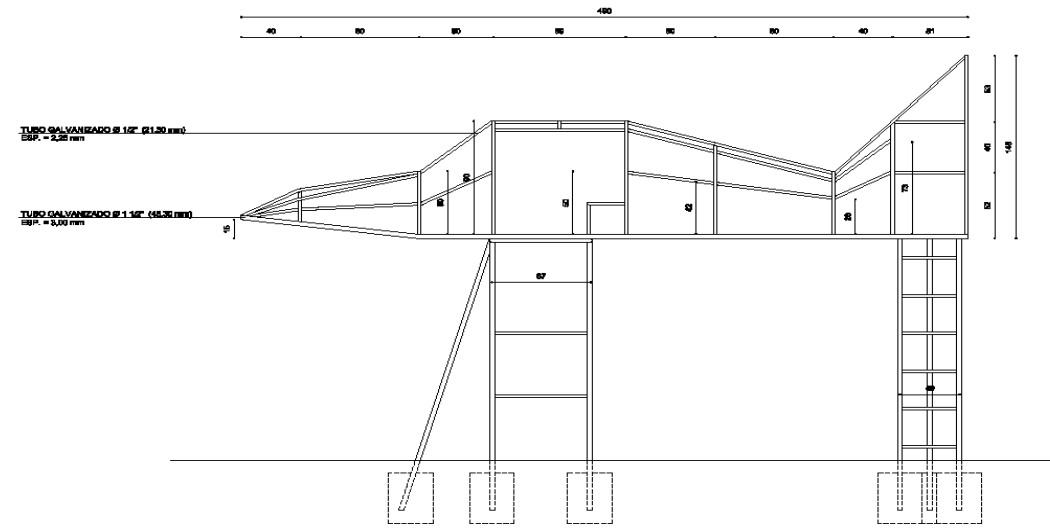
VISTA LATERAL
