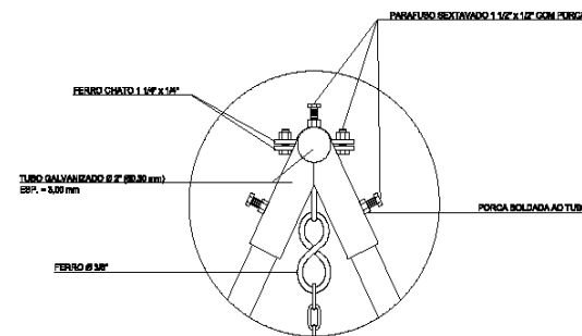
DETALHE 3 ESCALA 1:5
