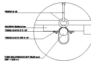
DETALHE 1 ESCALA 1:5
