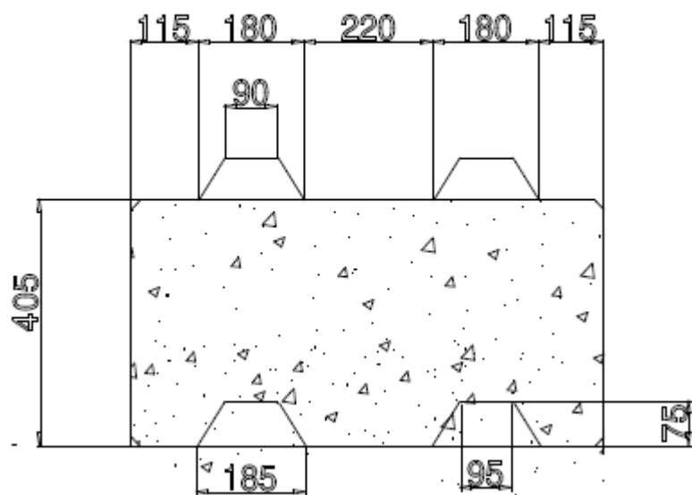
Corte A-A'
