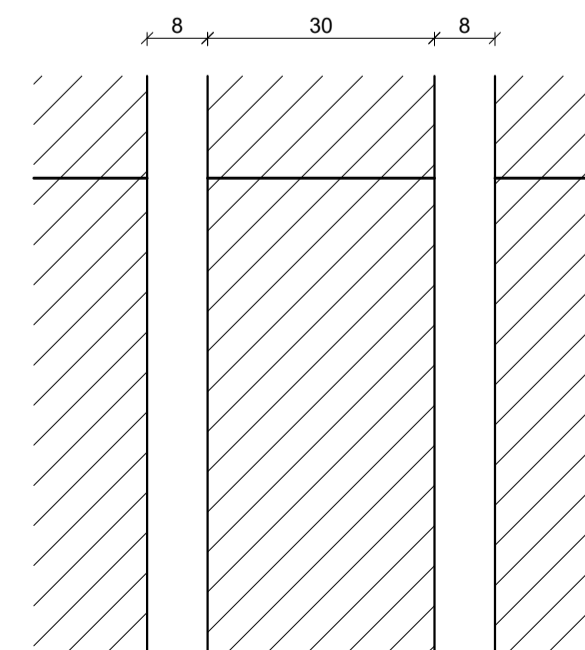
07 DET. 02 ESCALA: 1:10
