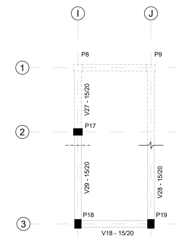
05 LOCAÇÃO PILARES 1,70 m ESCALA: 1:50
